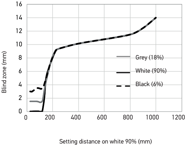
S3N-PR-*-M01-* (Blind zone)
