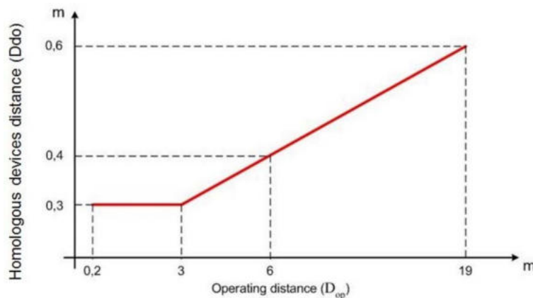
Fig 16 - ESPE Type2
