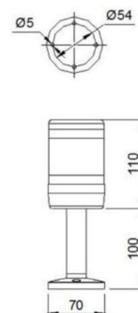
Fig 108 - Module SU-LMS-1B + LMS-1
