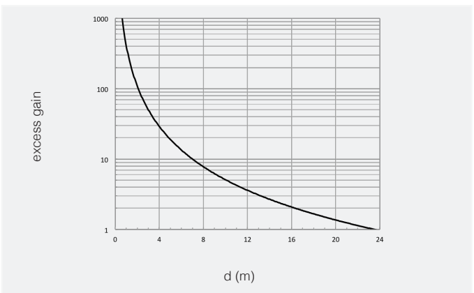
MVE/**-**- MVR/**-**- parallel displacement
