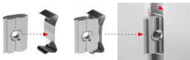
Пазовые сухари, поворотнo-вставные, для крепления VESA АТРН-IP
