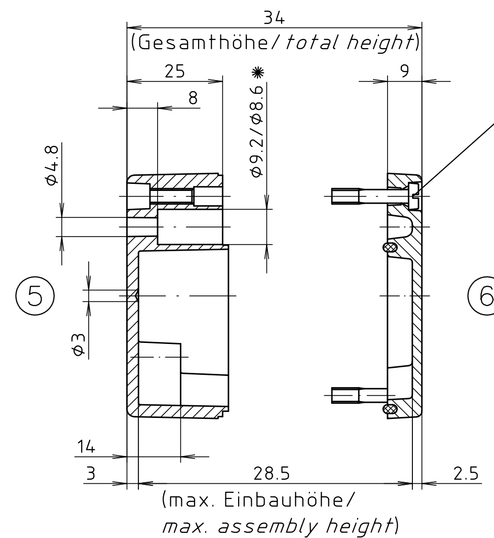
Zylinderschraube M4 x 20/7 ähnl. DIN EN ISO 1207/ cylinder screw M4 x 20/7 similar to DIN EN ISO 1207
