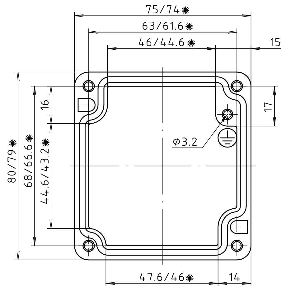
Deckel/ lid
