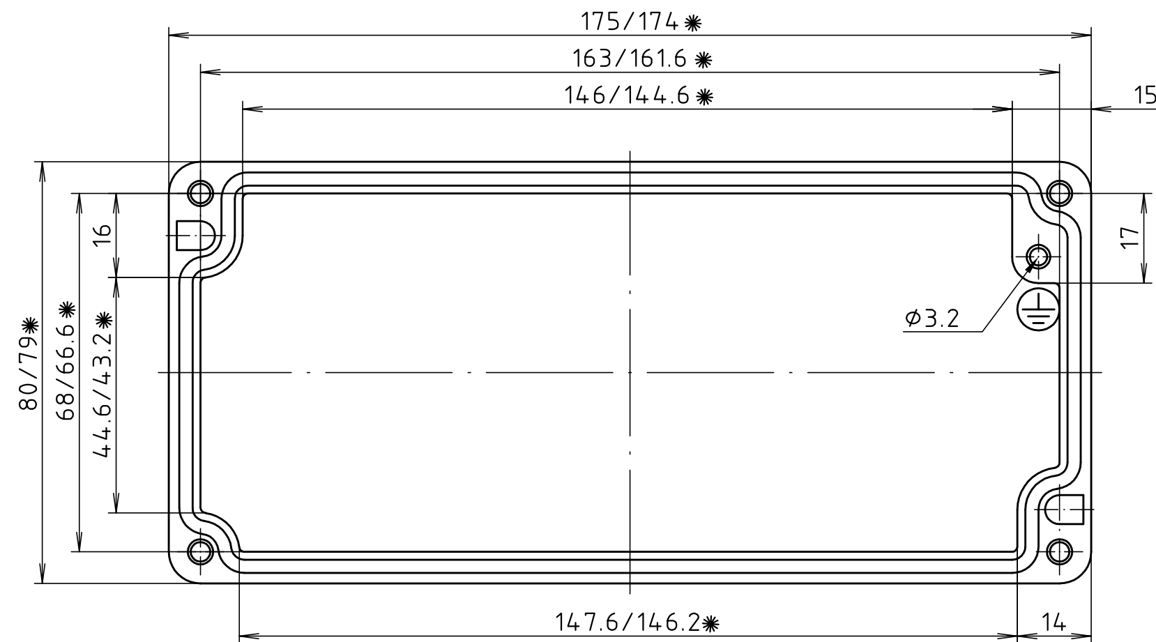
Deckel / lid
