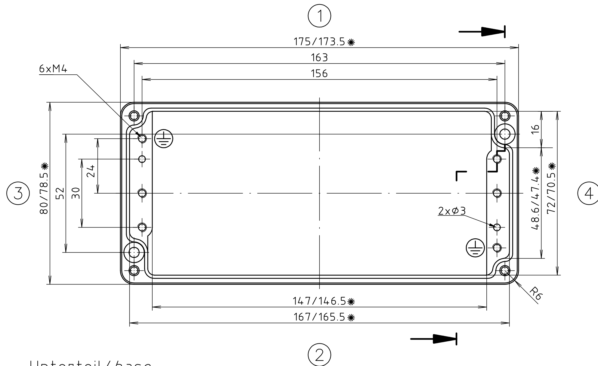
Unterteil / base
