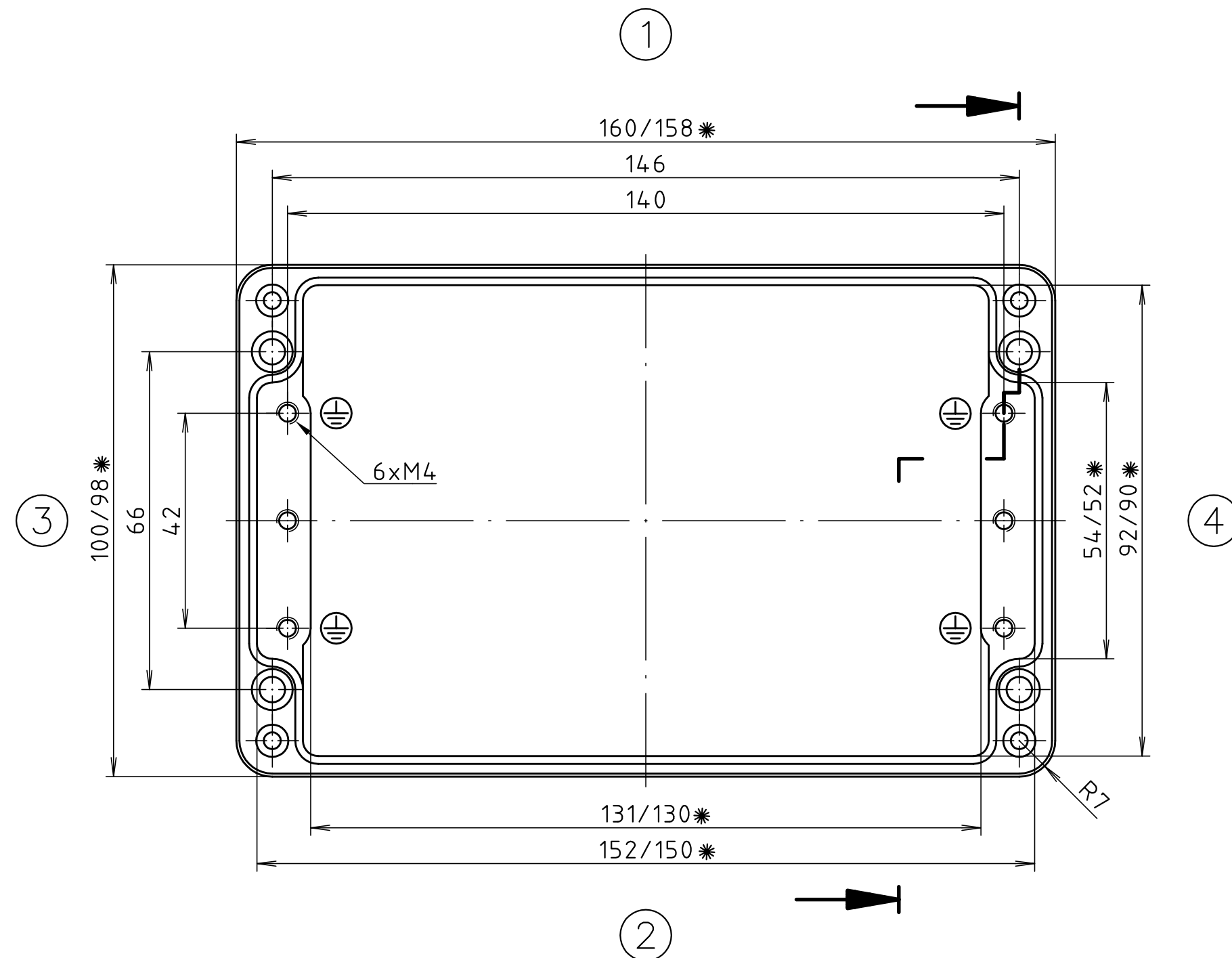
Unterteil / base
