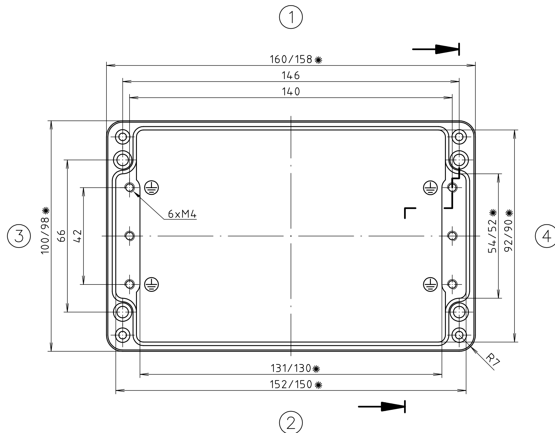
Unterteil / base
