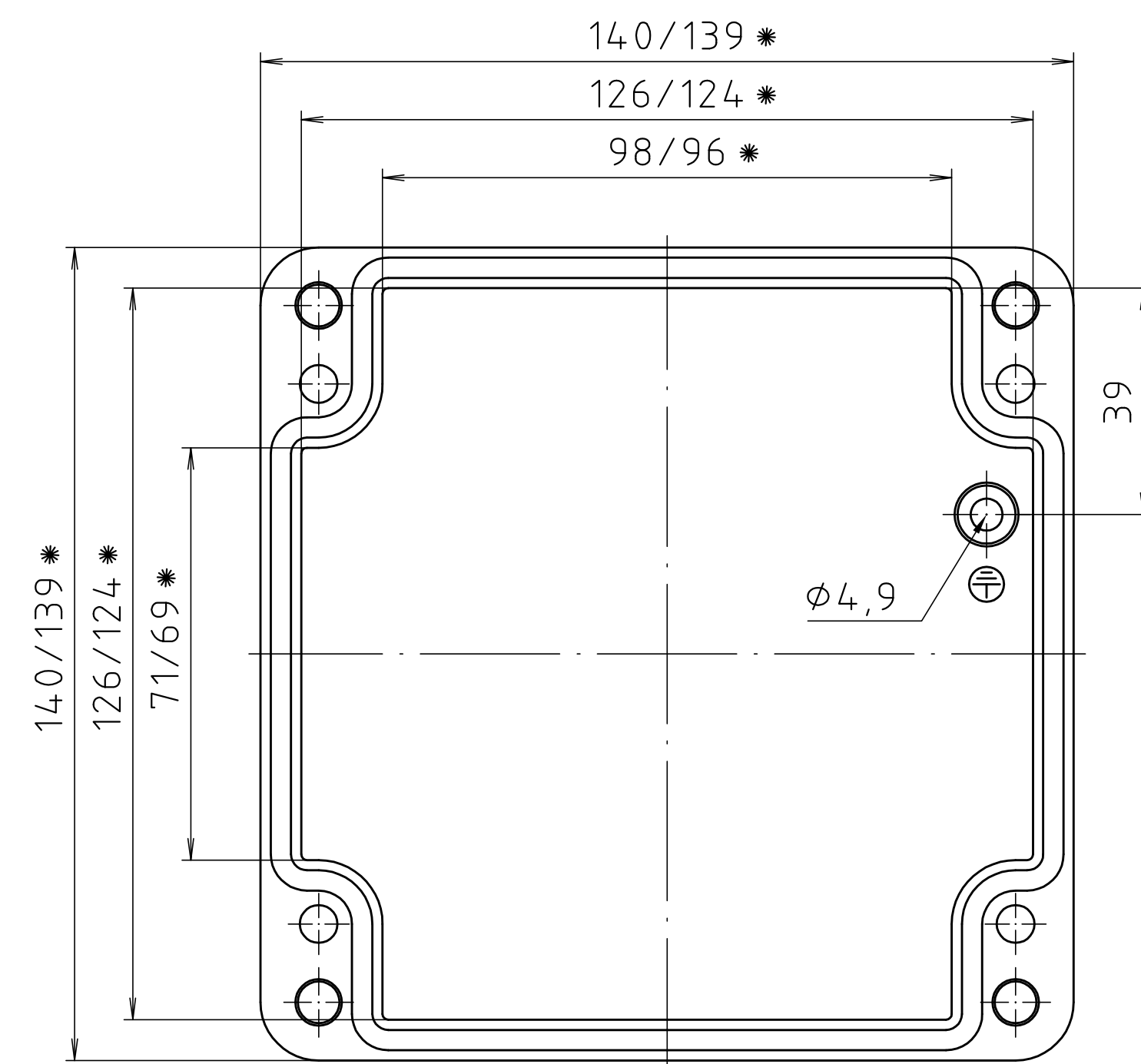
Deckel/ lid
