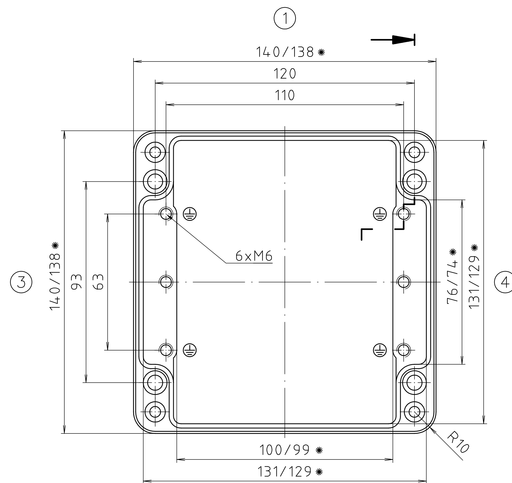
Unterteil/ base
