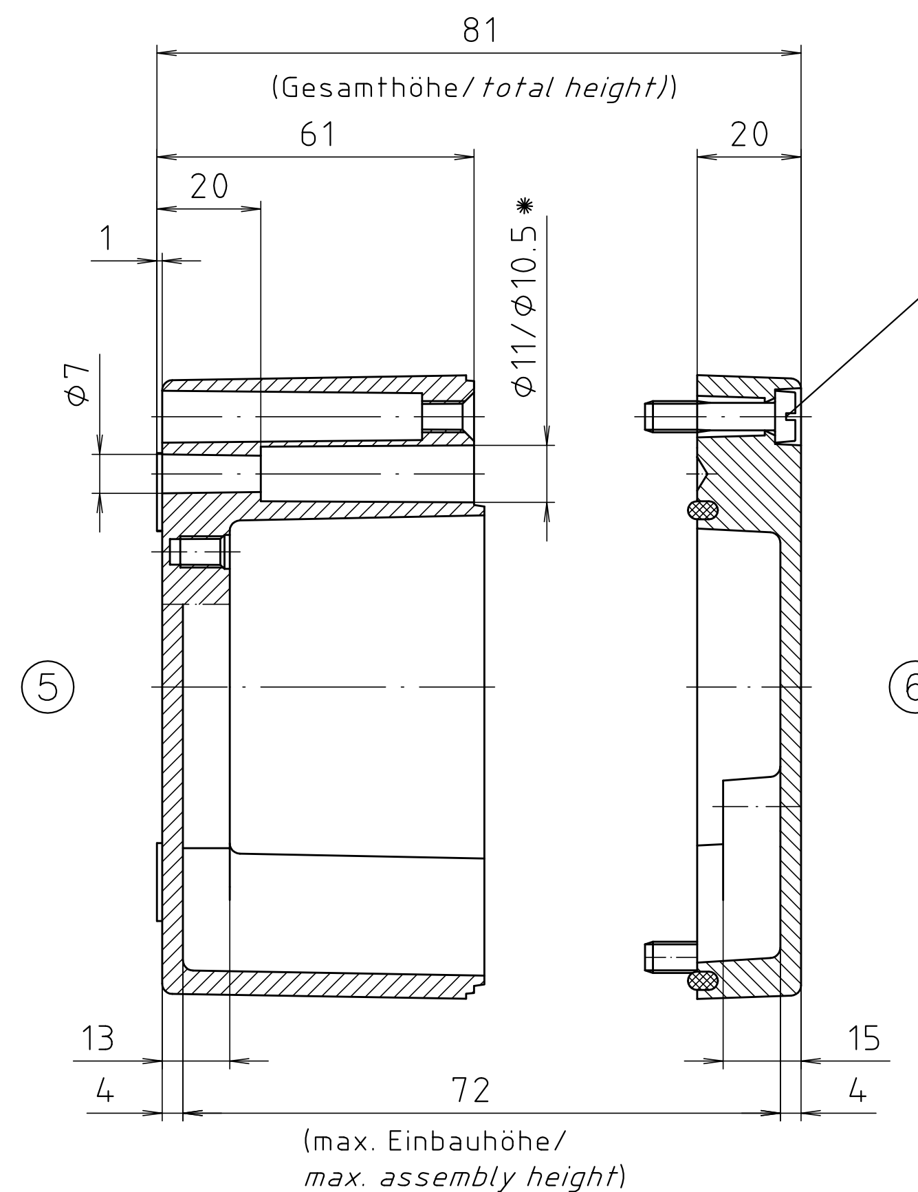
Zylinderschraube M6 x 25/10 ähnl. DIN EN ISO 1207/ cylinder screw M6 x 25/10 similar to DIN EN ISO 1207
