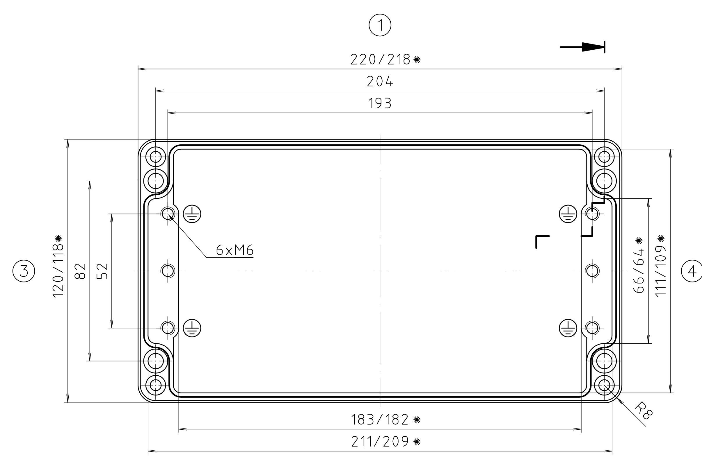
Unterteil/ base
