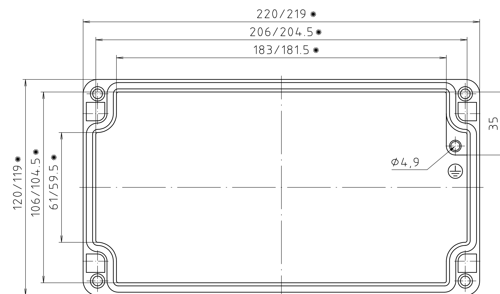
Deckel/ lid
