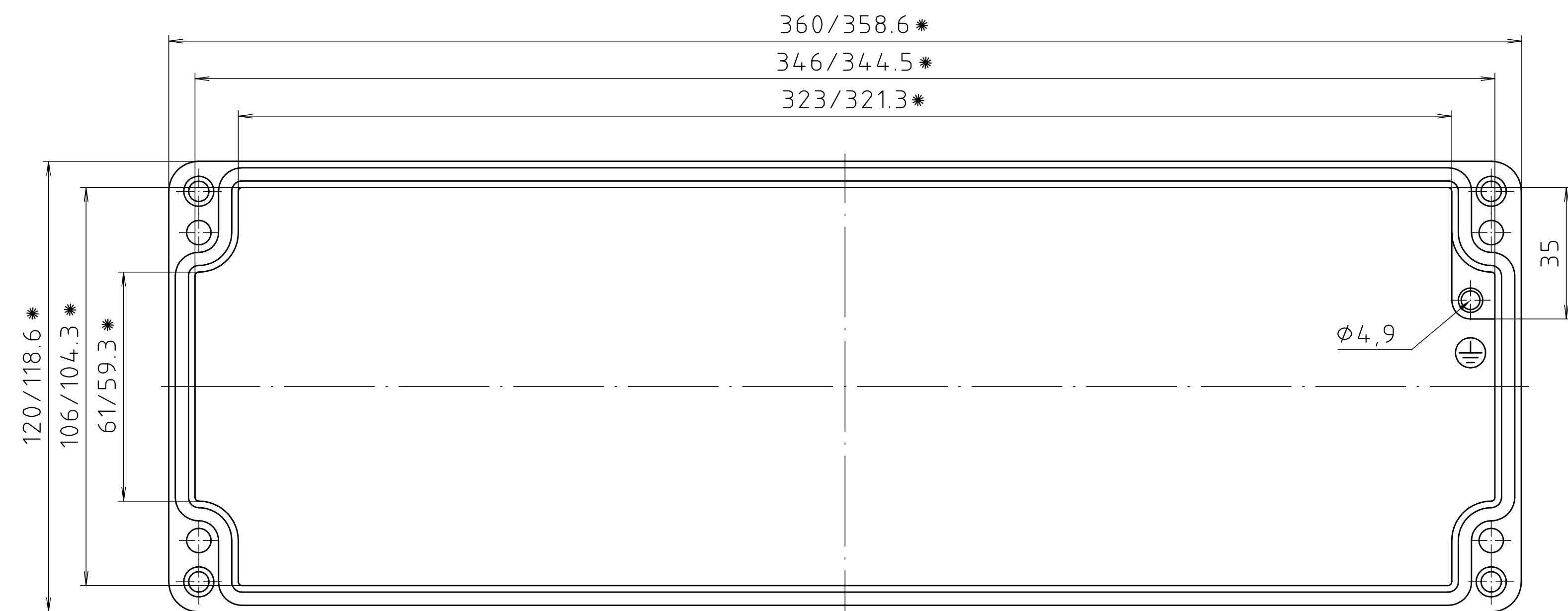
Deckel / lid
