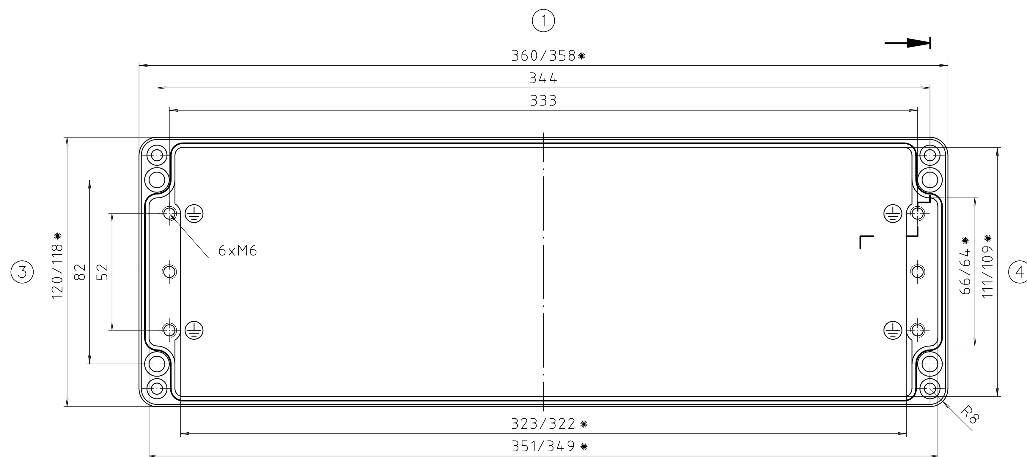
Unterteil / base
