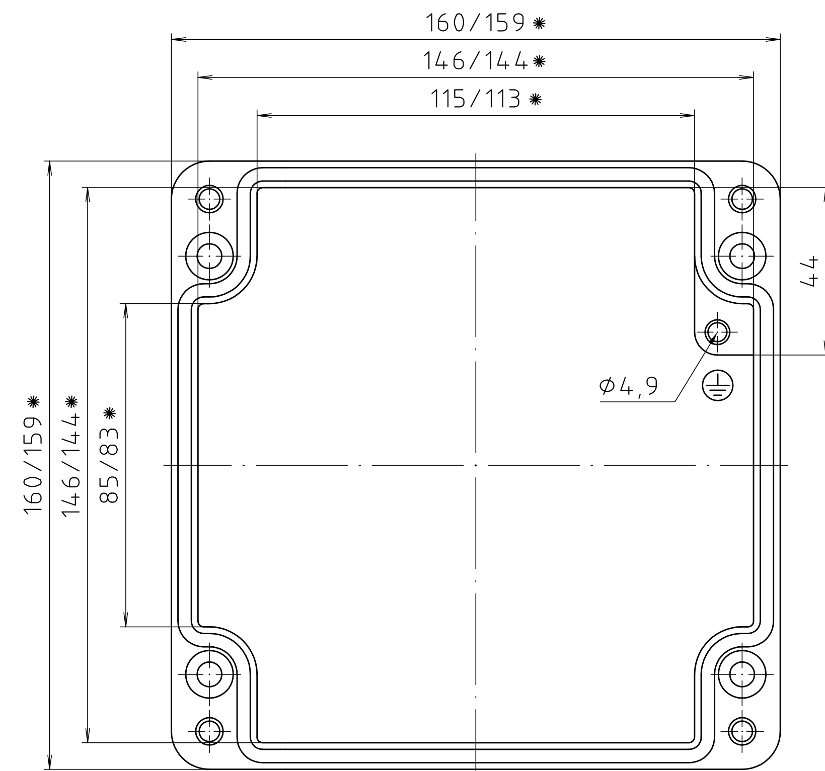
Deckel / lid
