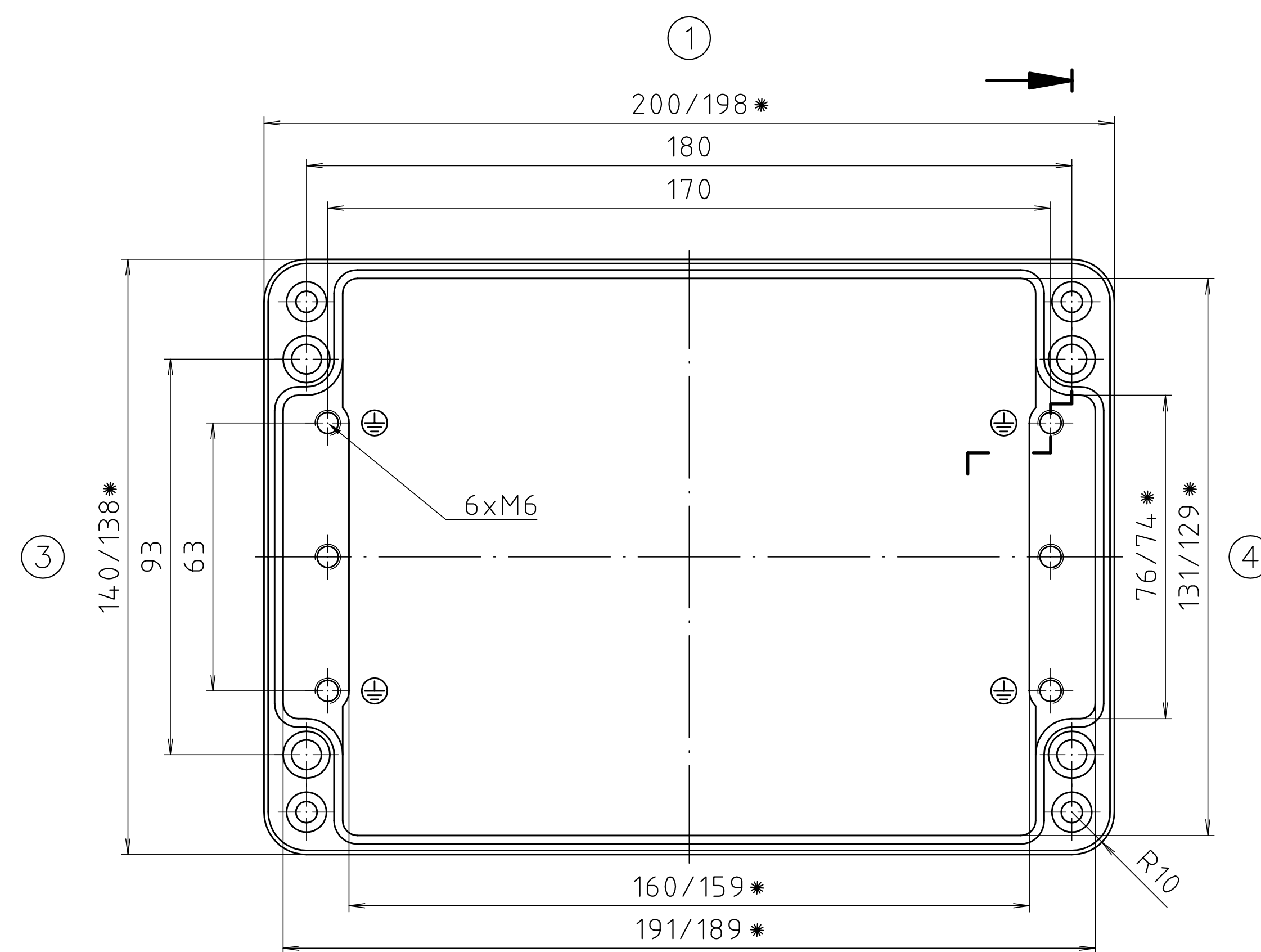
Unterteil / base
