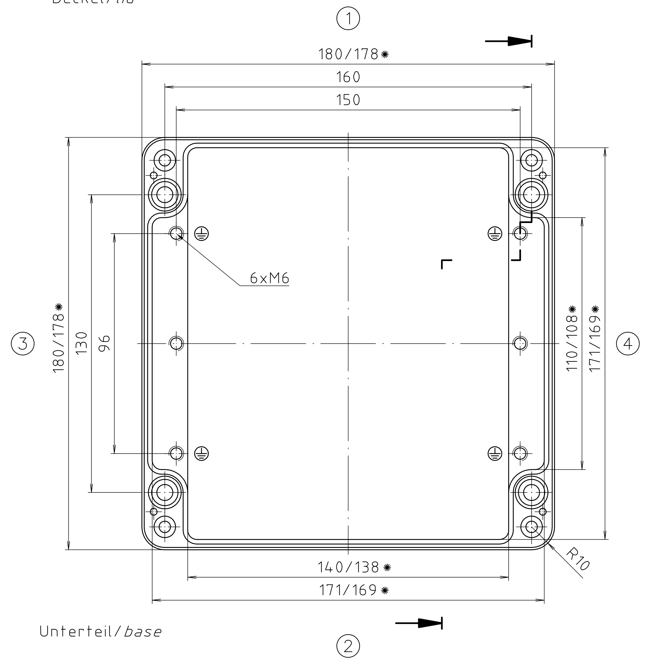
Deckel / lid
