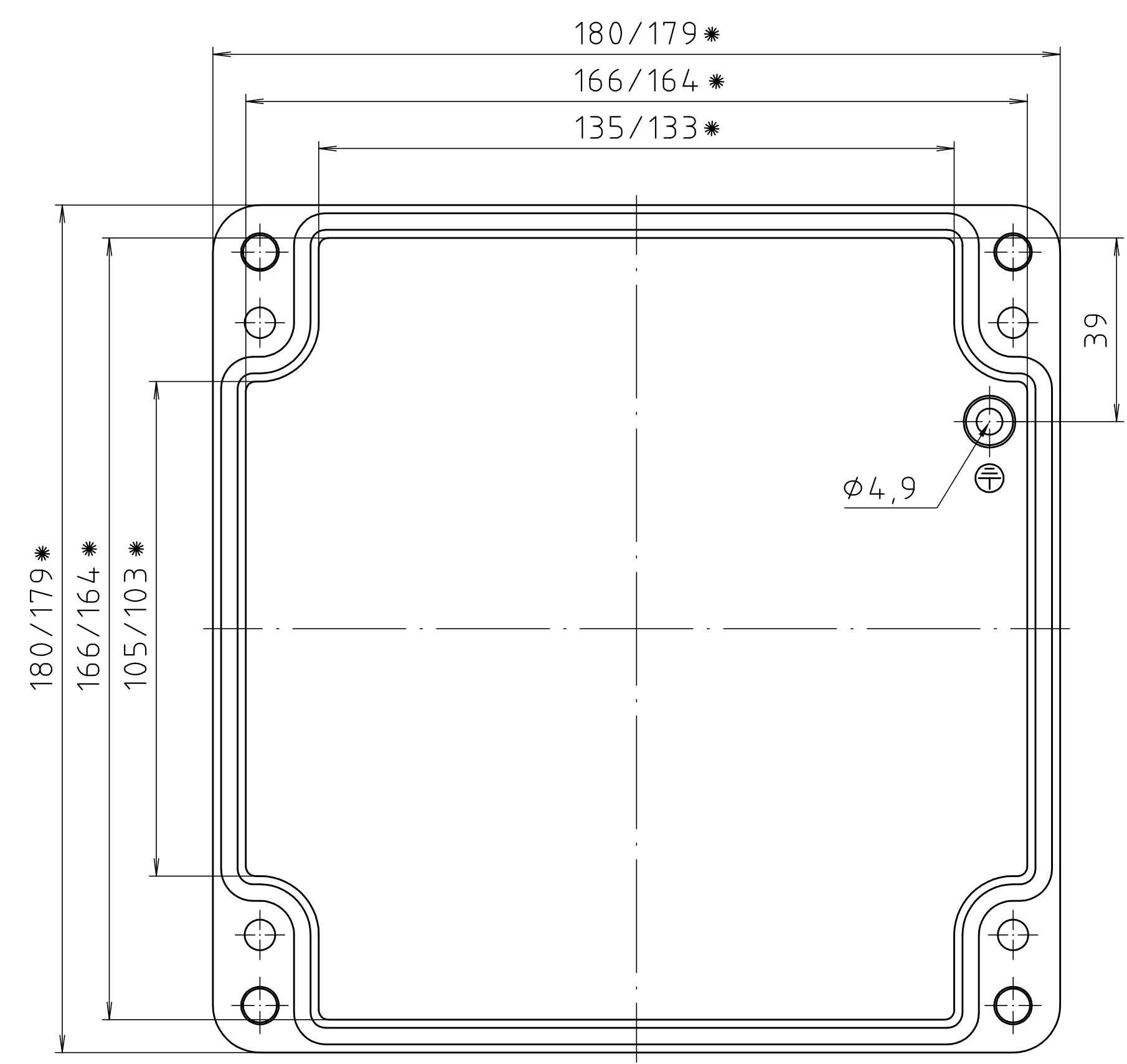
Deckel / lid
