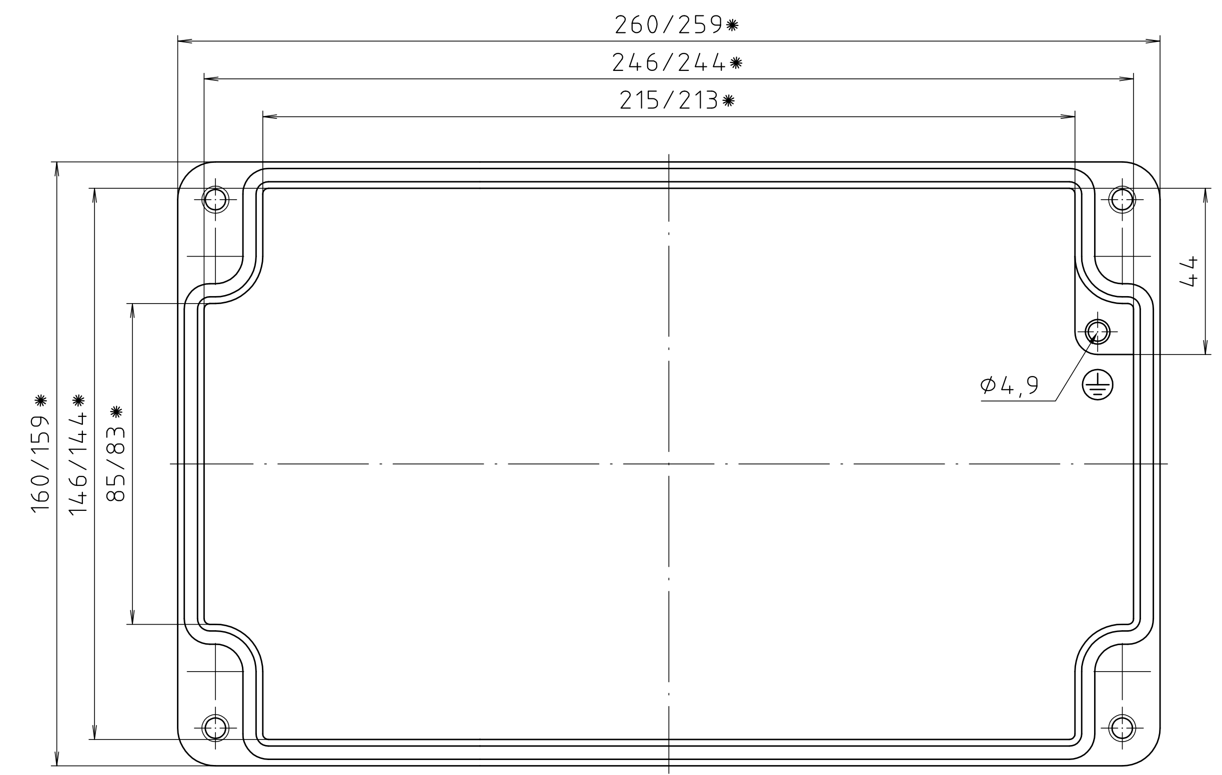
Deckel/ lid
