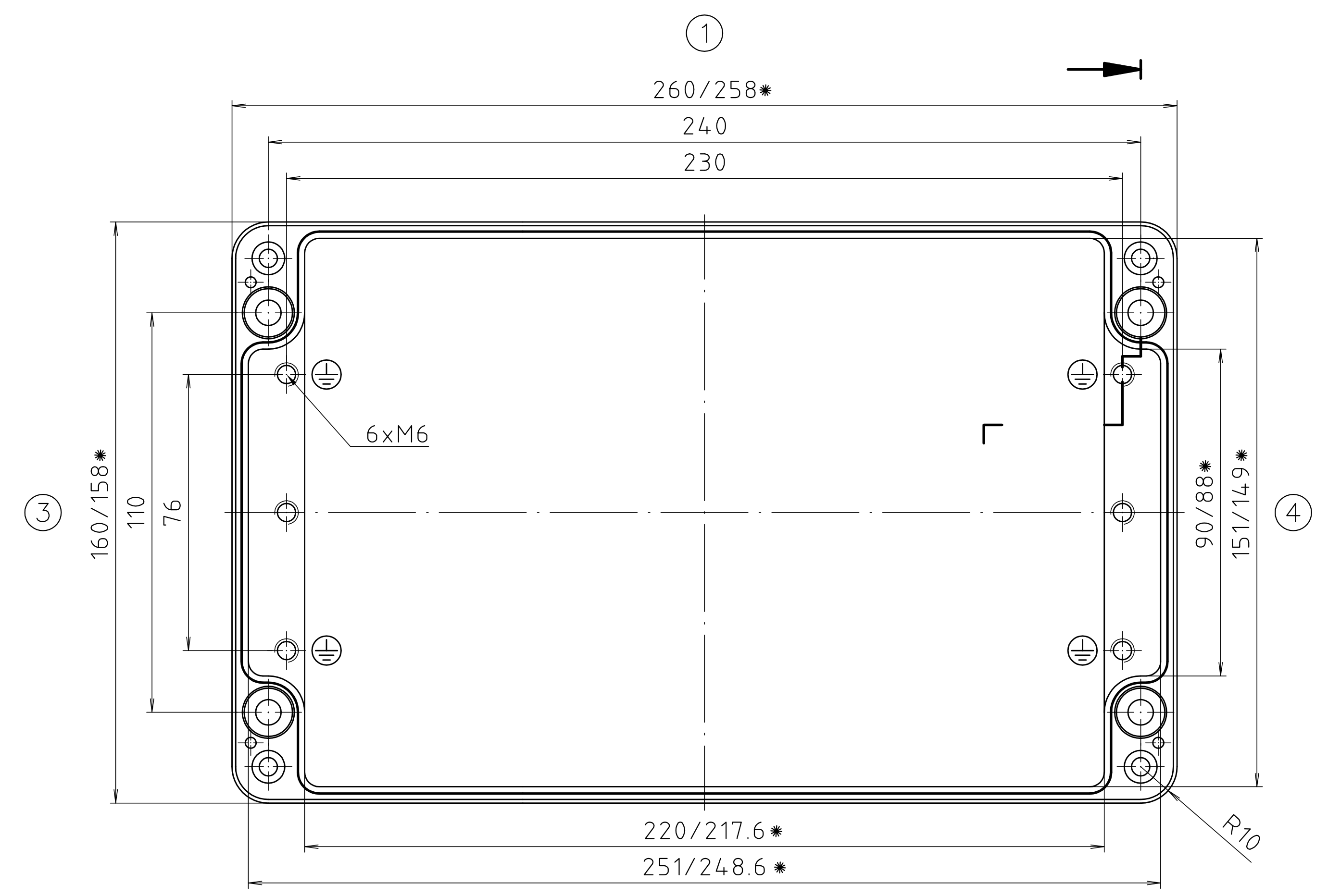
Unterteil/ base
