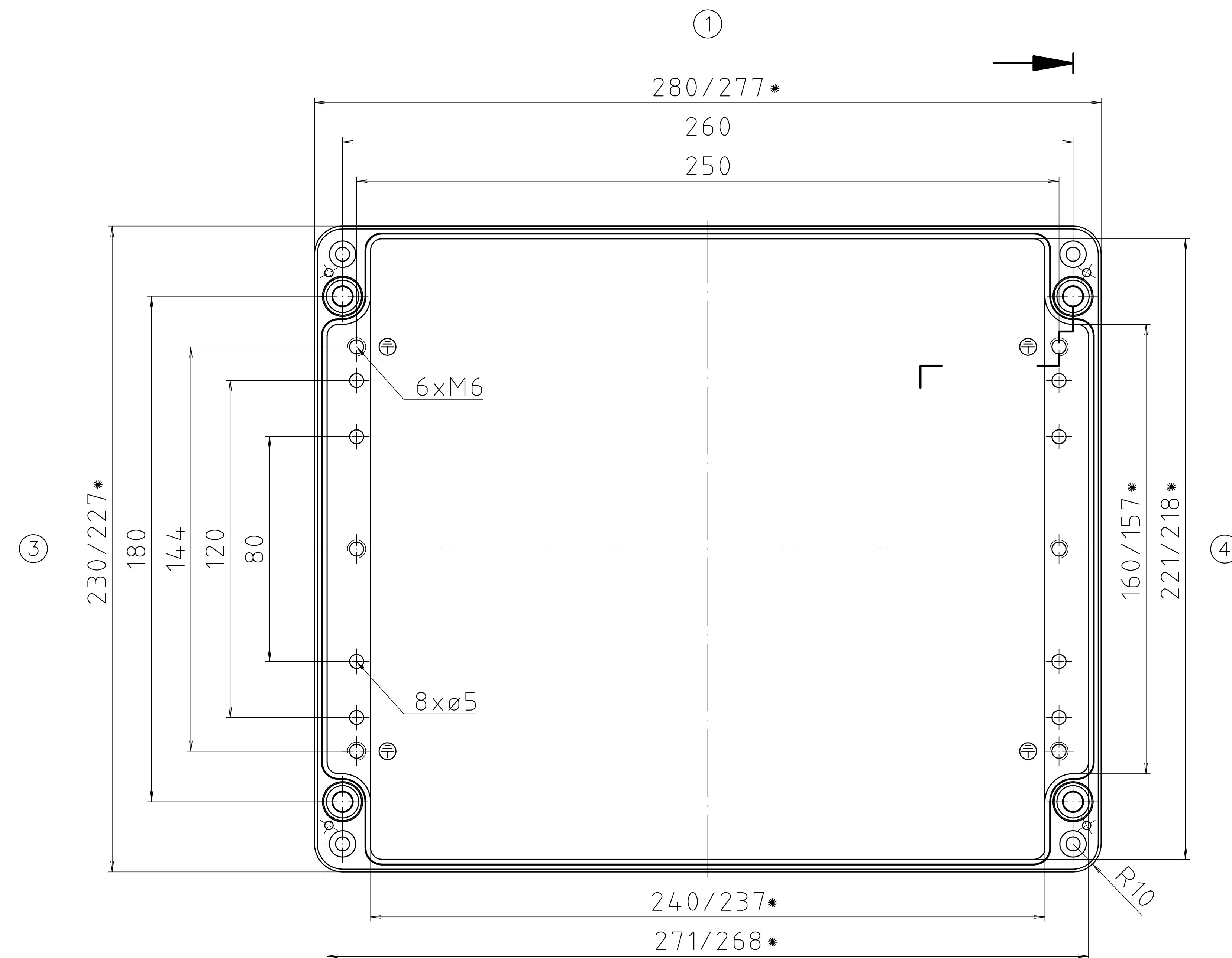
Deckel / lid
