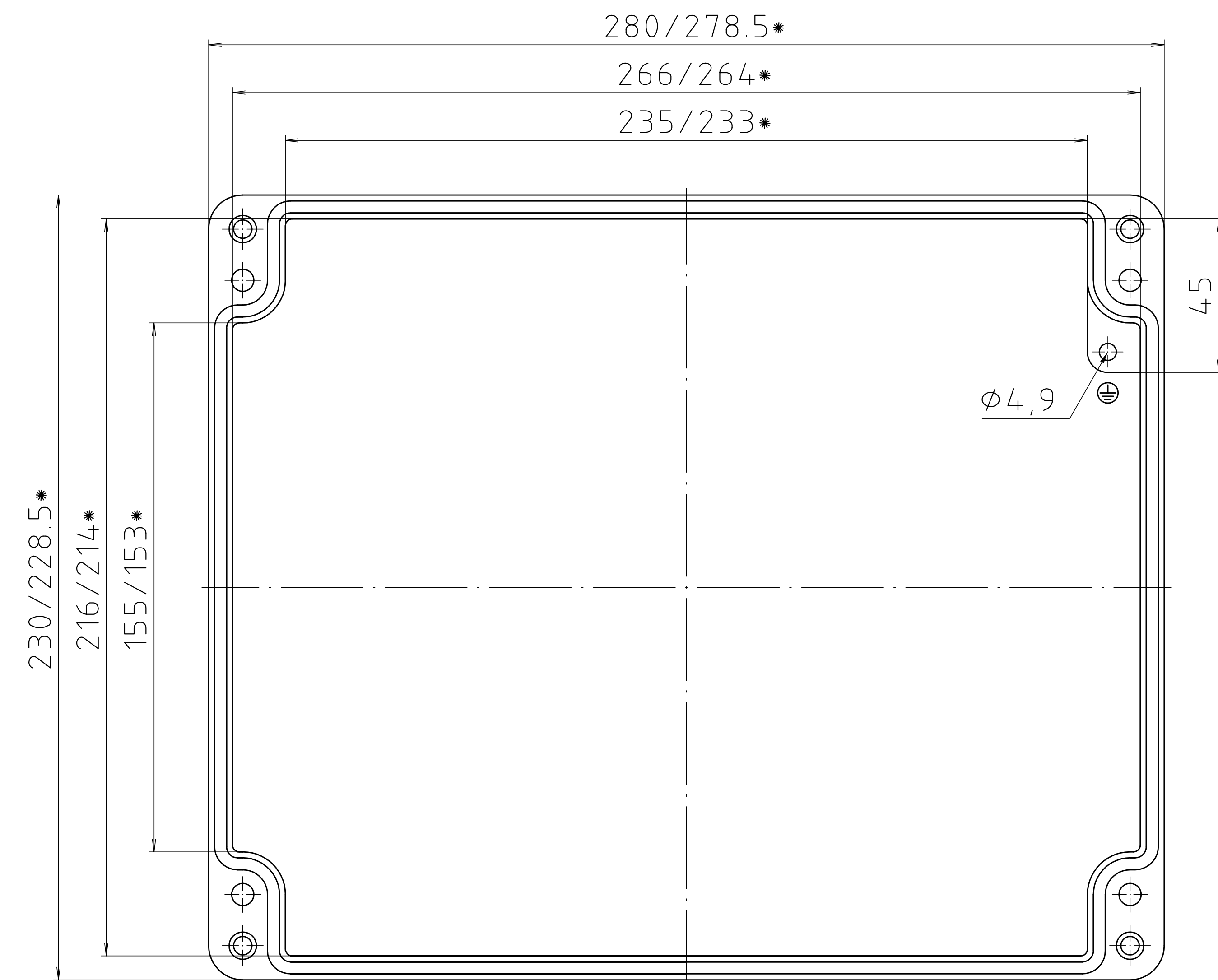
Deckel / lid
