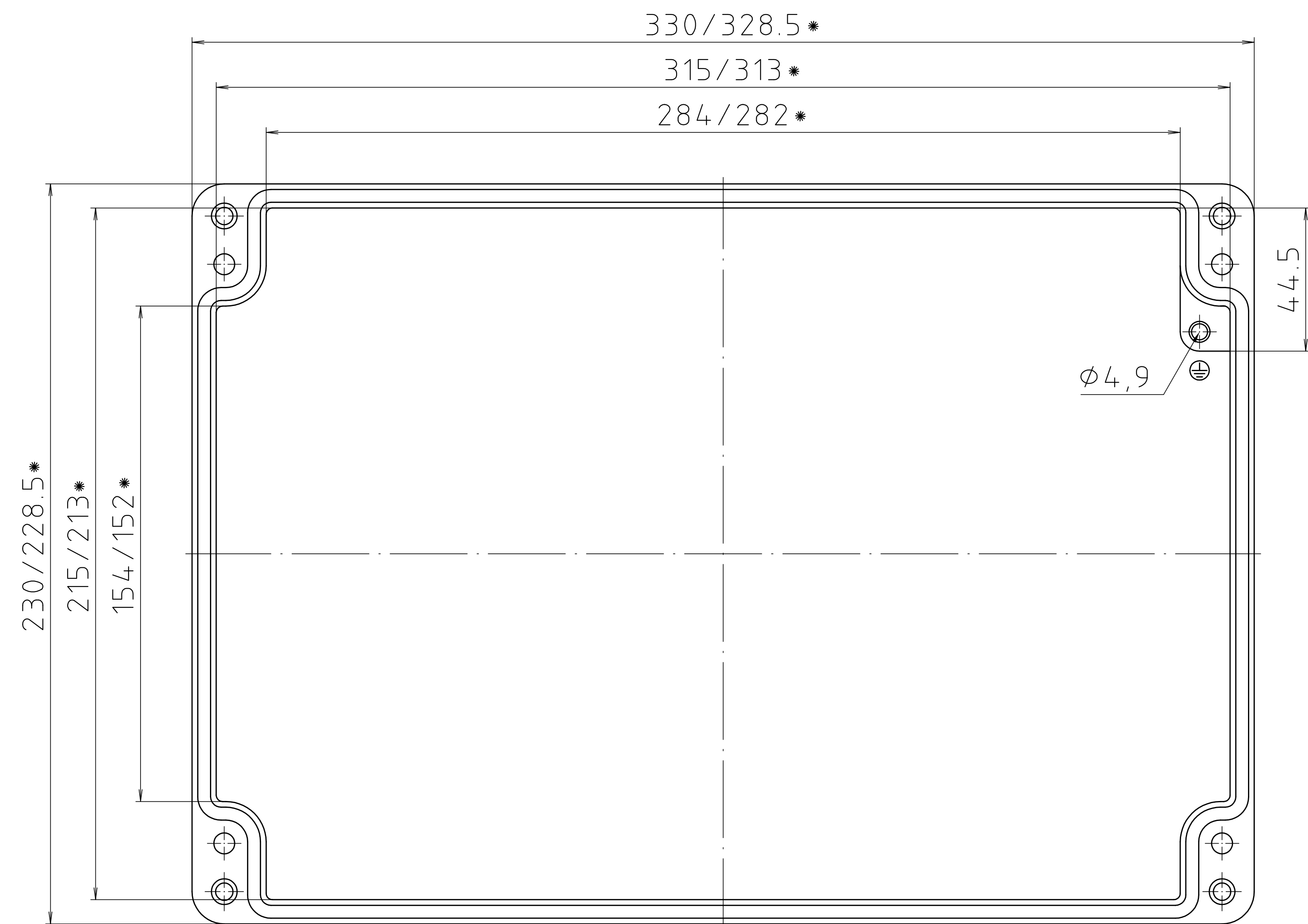
Deckel/ lid
