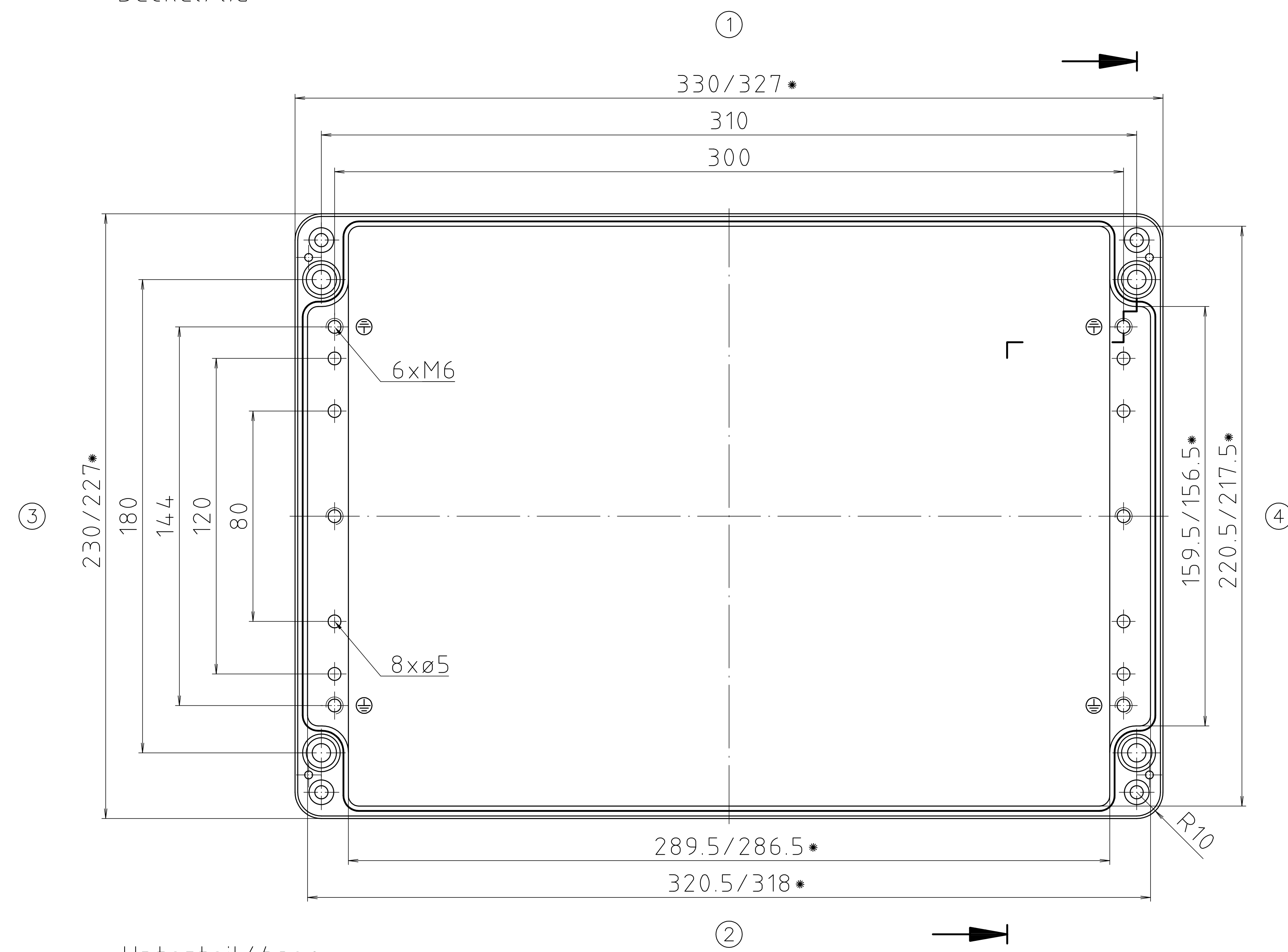
Unterteil/ base
