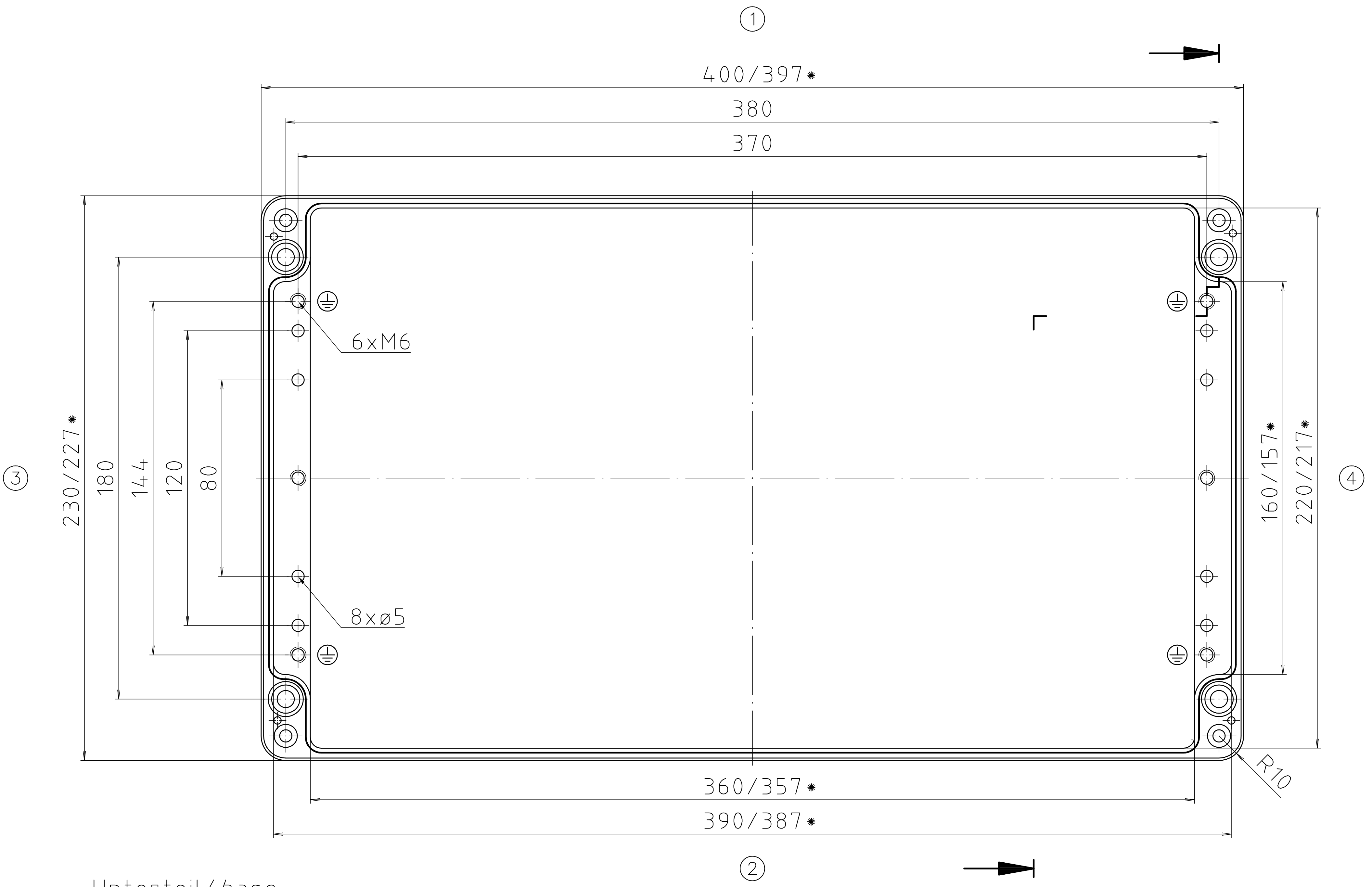
Unterteil/base
