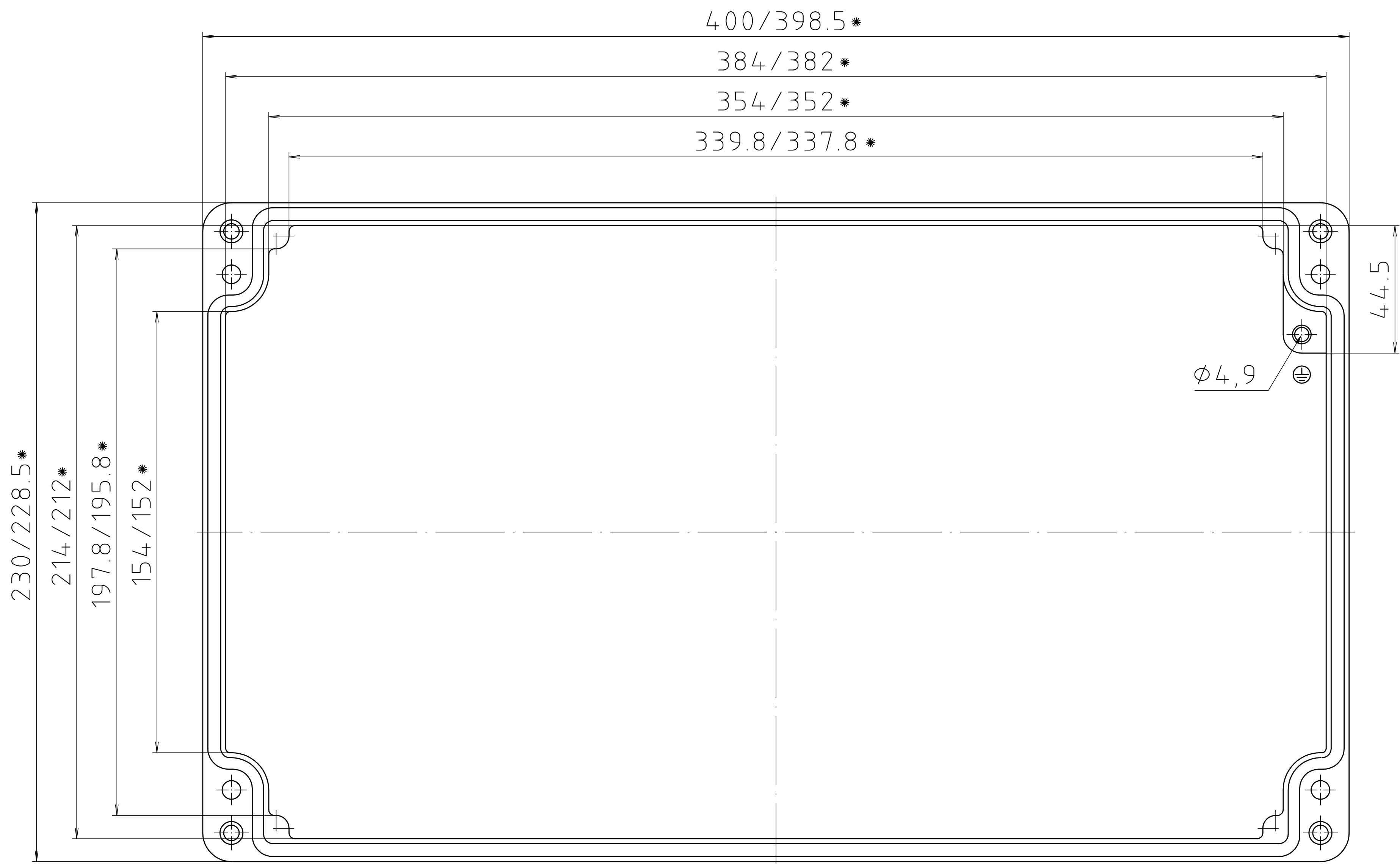
Deckel/ lid
