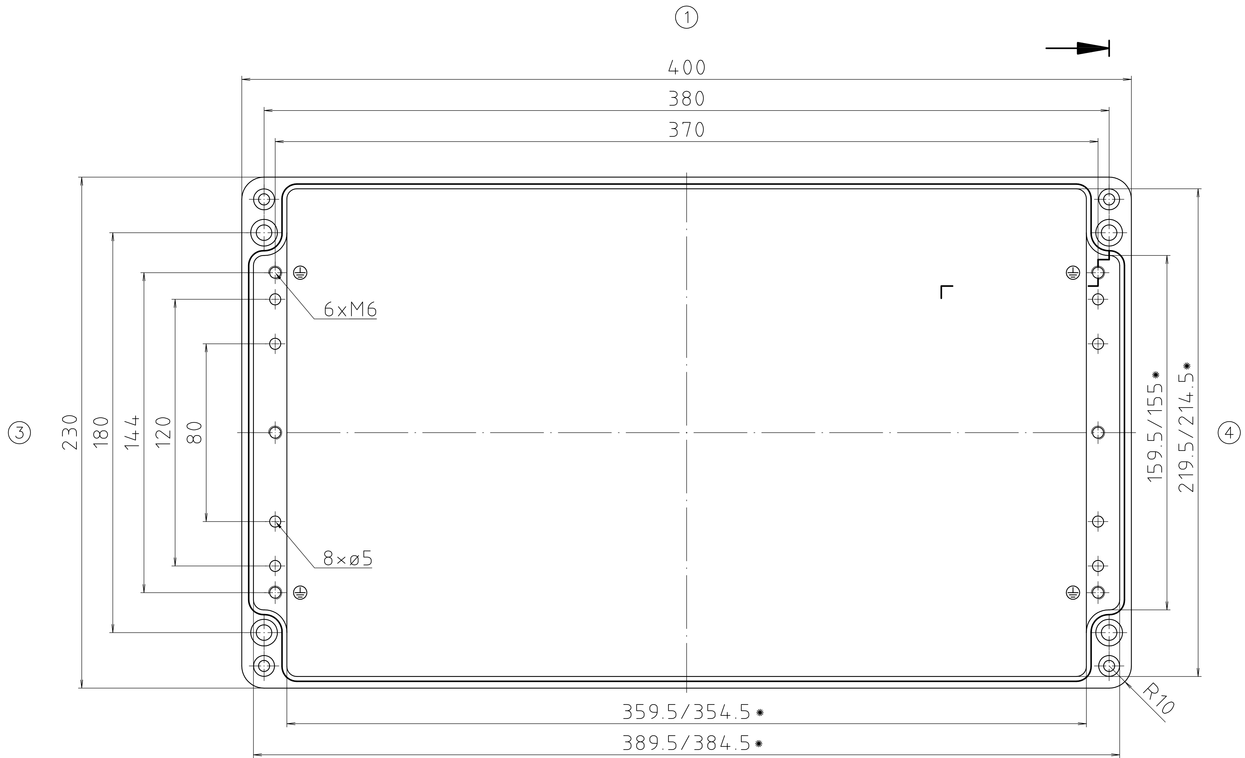
Deckel/ lid
