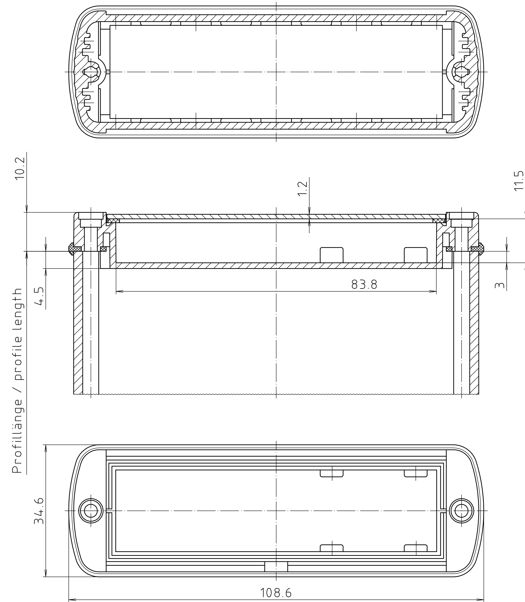
Ansicht ohne Profilkappe bzw. ohne Profilklappe View without profile lid resp. profile shutter
