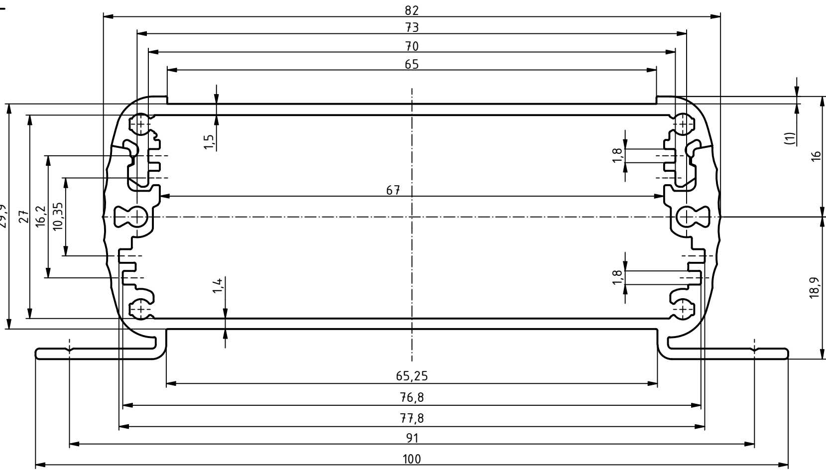
ABPH 800 WL
