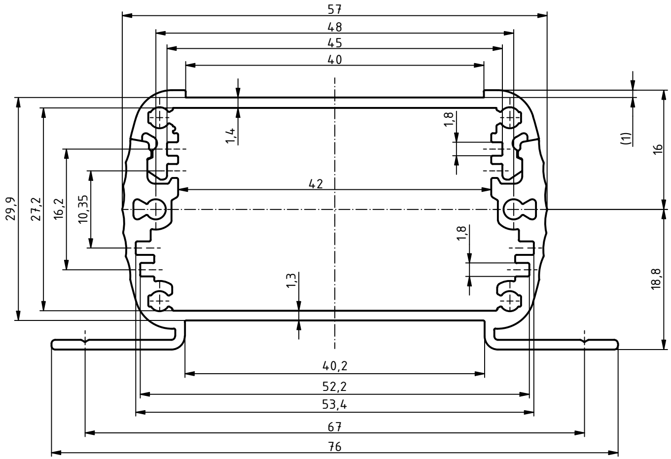
ABPH 600 WL
