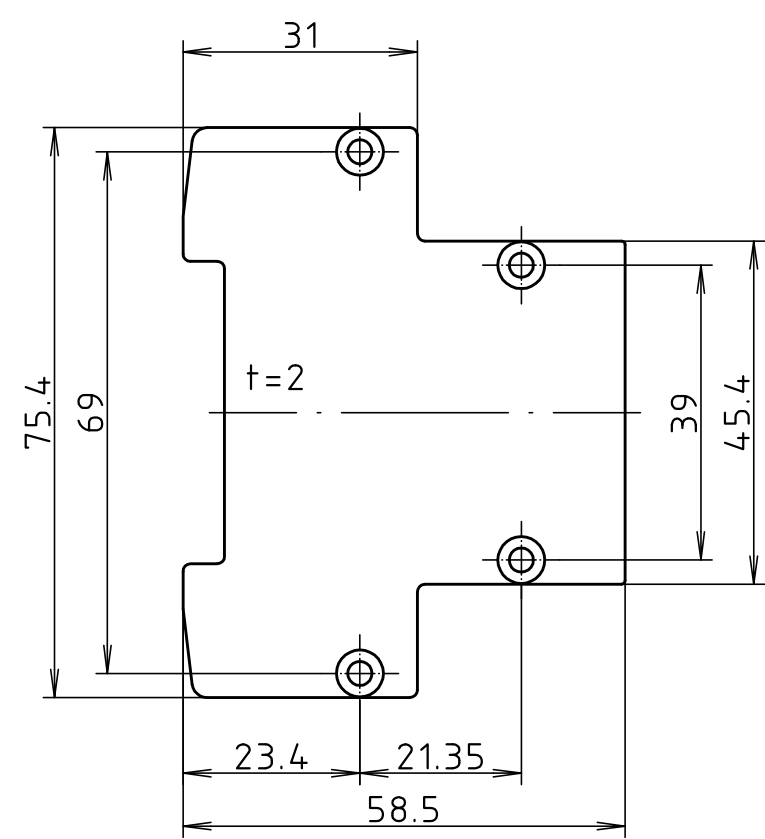
AR 75/45-KS-AL
