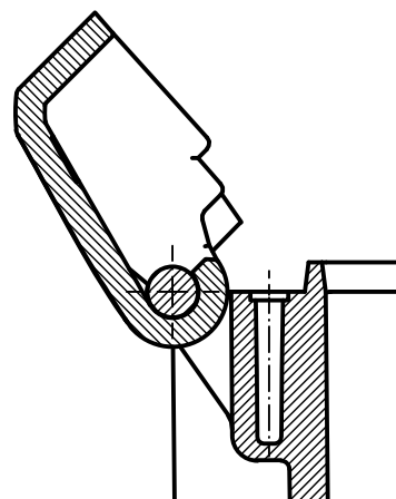
B SC montiert B SC mounted
