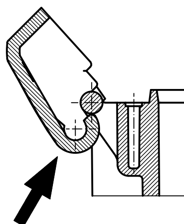
B SC montiert B SC mounted
