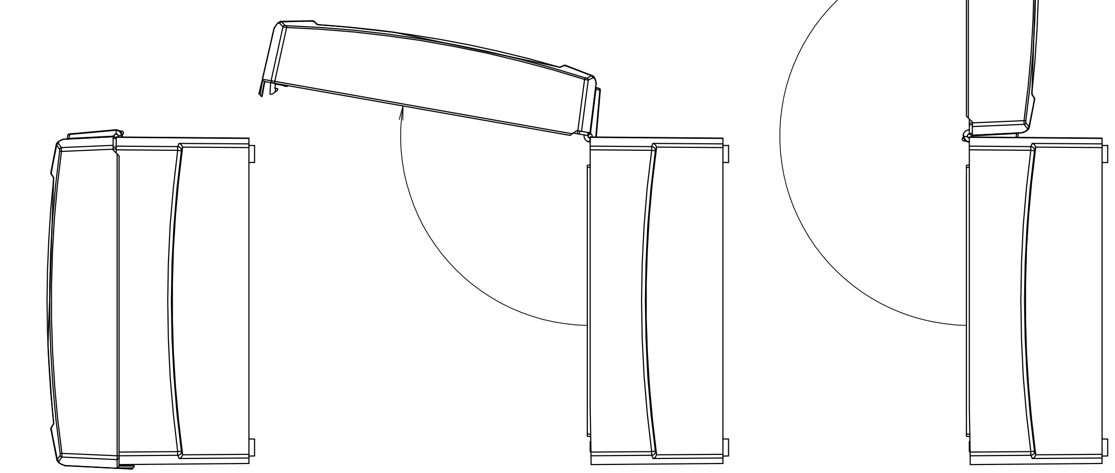
Gehäuse geschlossen Enclosure closed 1. Rastpunkt über 90° 1st notch over 90° Gehäuse offen über 180° Enclosure open over 180°
