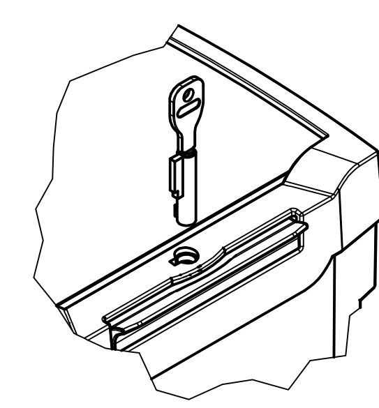
Schloss SHL0402 ( Zubehör ) Lock SHLO 402 ( accessory )
