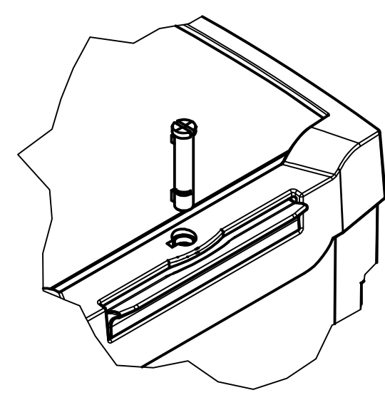
BCD-Sperrerr ( im Lieferumfang ) BCD catch ( included )
