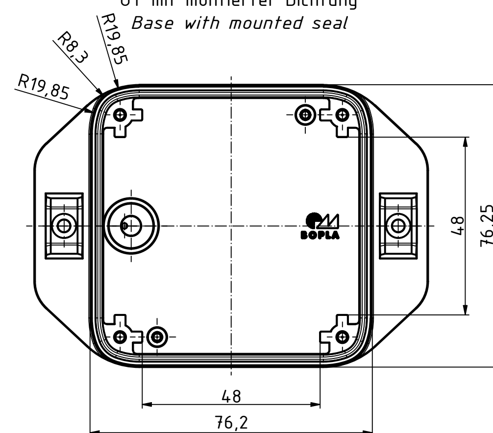
UT mit montierter Dichtung Base with mounted seal
