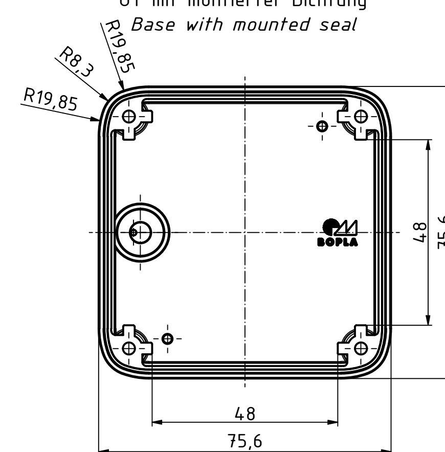
UT mit montierter Dichtung Base with mounted seal
