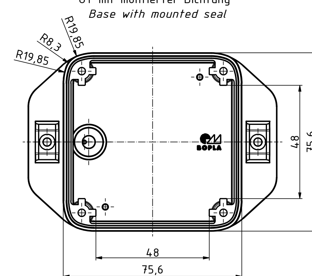
UT mit montierter Dichtung Base with mounted seal
