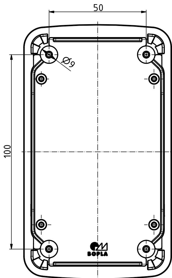
OT mit montierter Dichtung Lid with mounted seal
