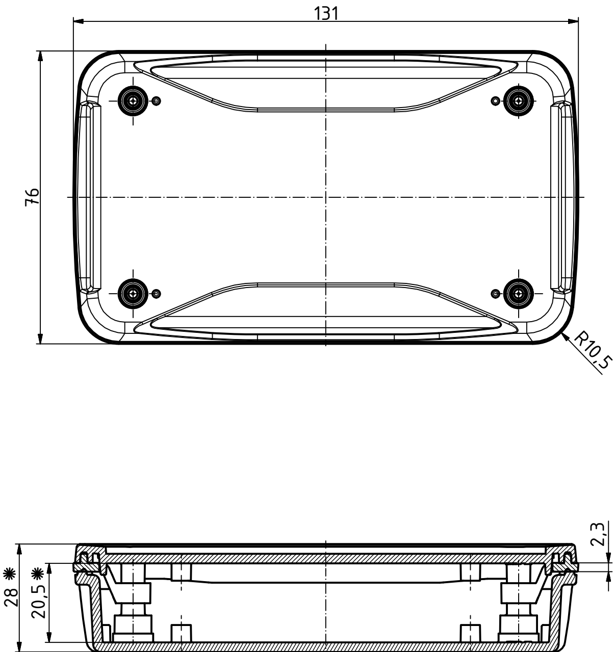
BOP 500 + BOP 500 DI
