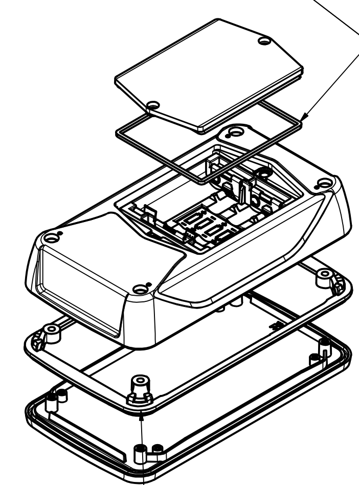
Gehäusedichtung Enclosure seal
