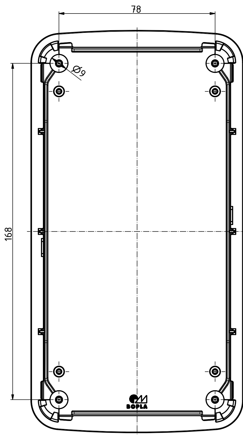
OT mit montierter Dichtung Lid with mounted seal
