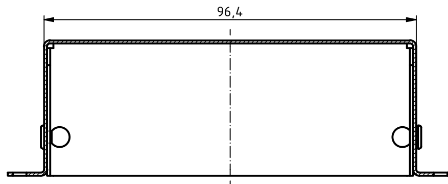
B-B ( 1 : 1 )
