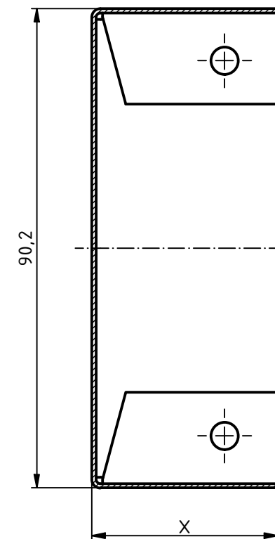
A-A ( 1 : 1 )
