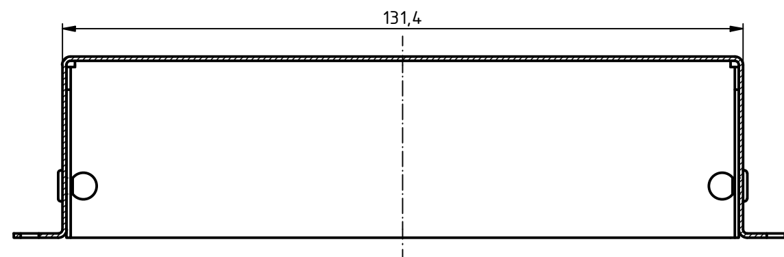
B-B ( 1 : 1 )
