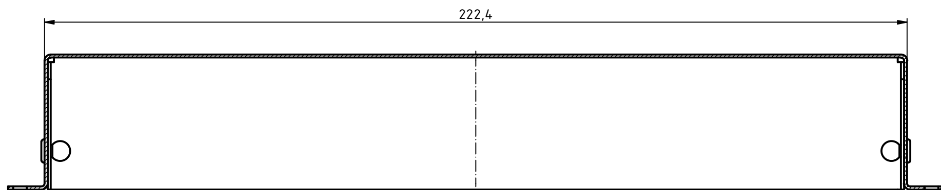
B-B ( 1 : 1 )
