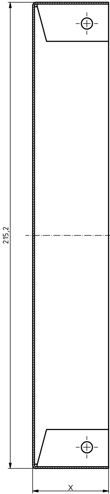
A-A ( 1 : 1 )
