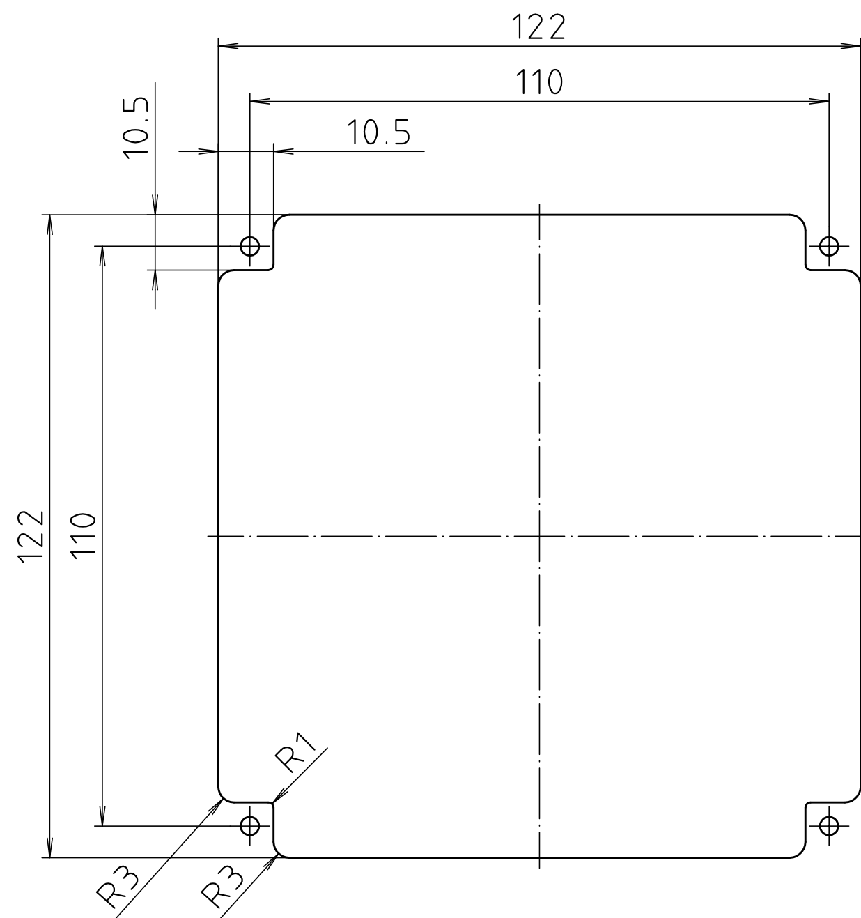
Schalttafelausschnitt/ panel cut-out
