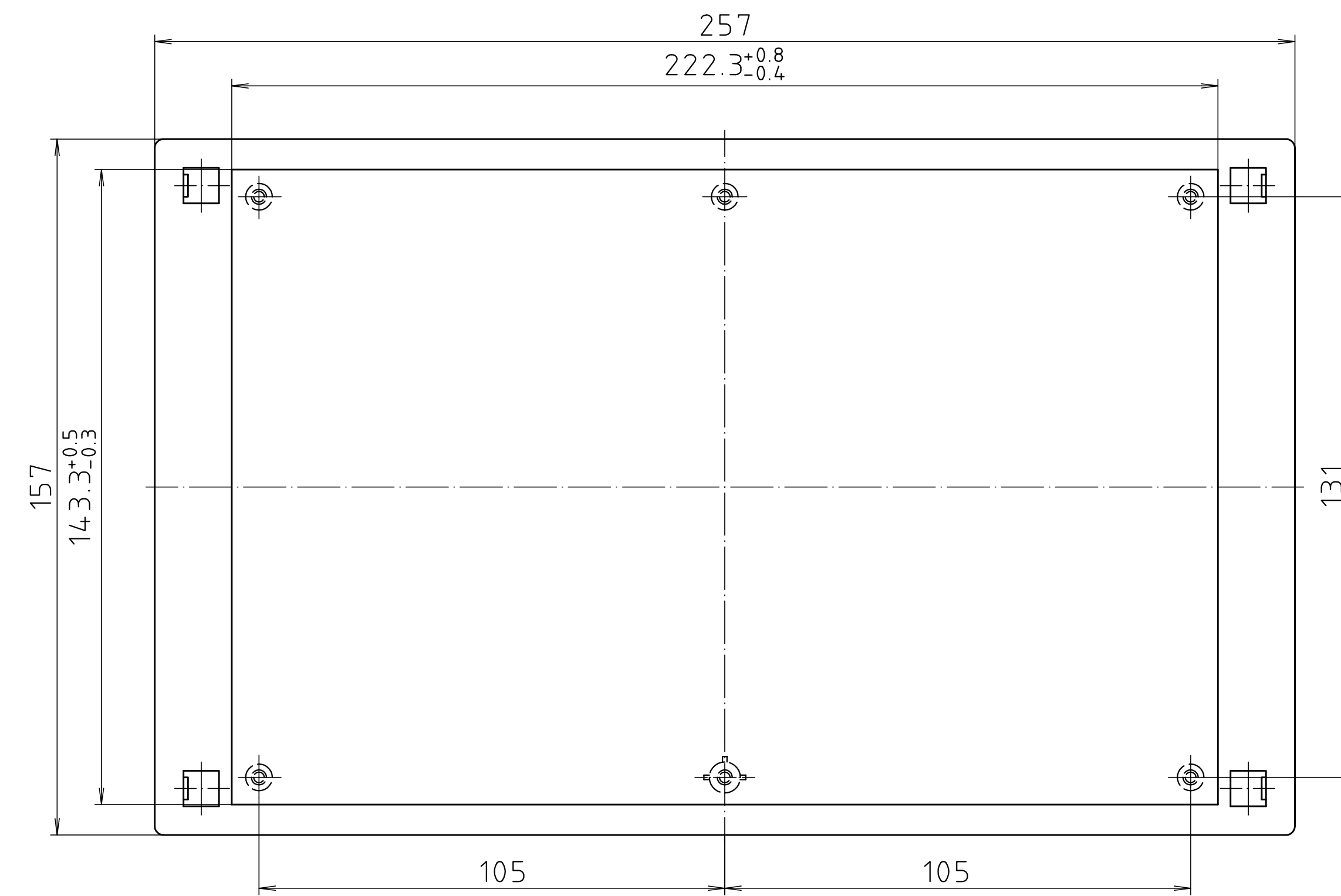
Schalttafelauausschnitt/ panel cut-out
