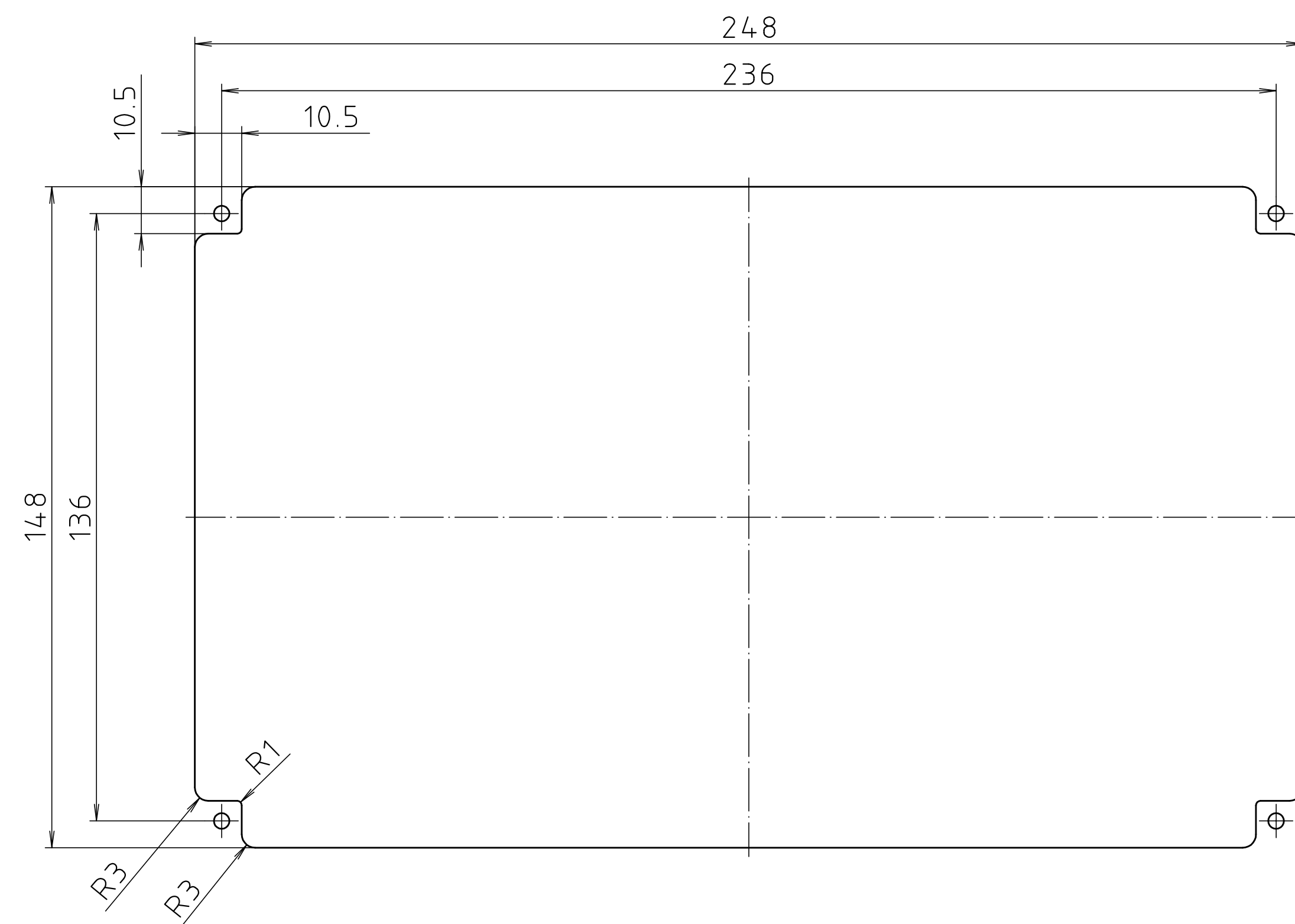
Schalttafelauausschnitt/ panel cut-out
