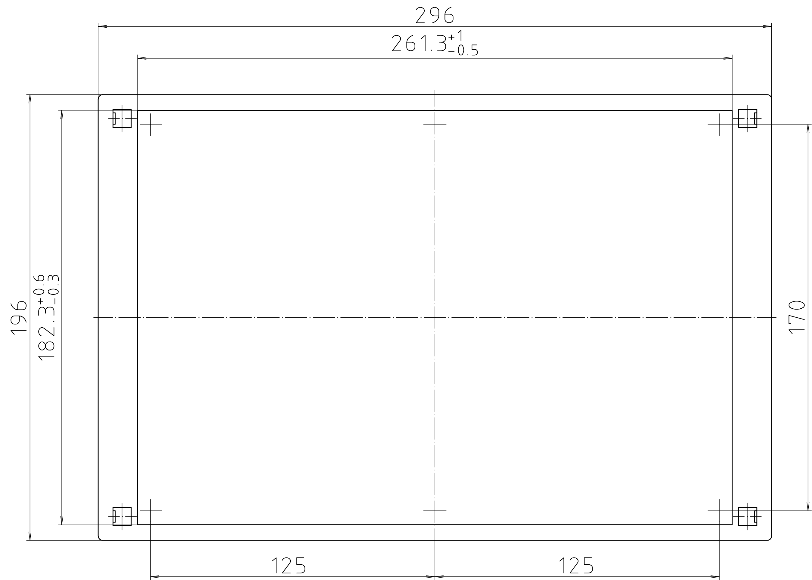
Schalttafelausschnitt/ panel cut-out
