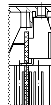
Anschlussklemme AK 700/. H/ Connection terminals AK 700/. H
