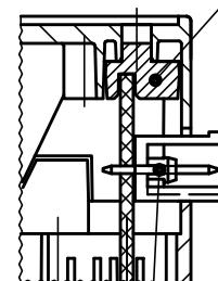
Stiftleiste STL 950/____ V/ pin bars STL 950/____ V
