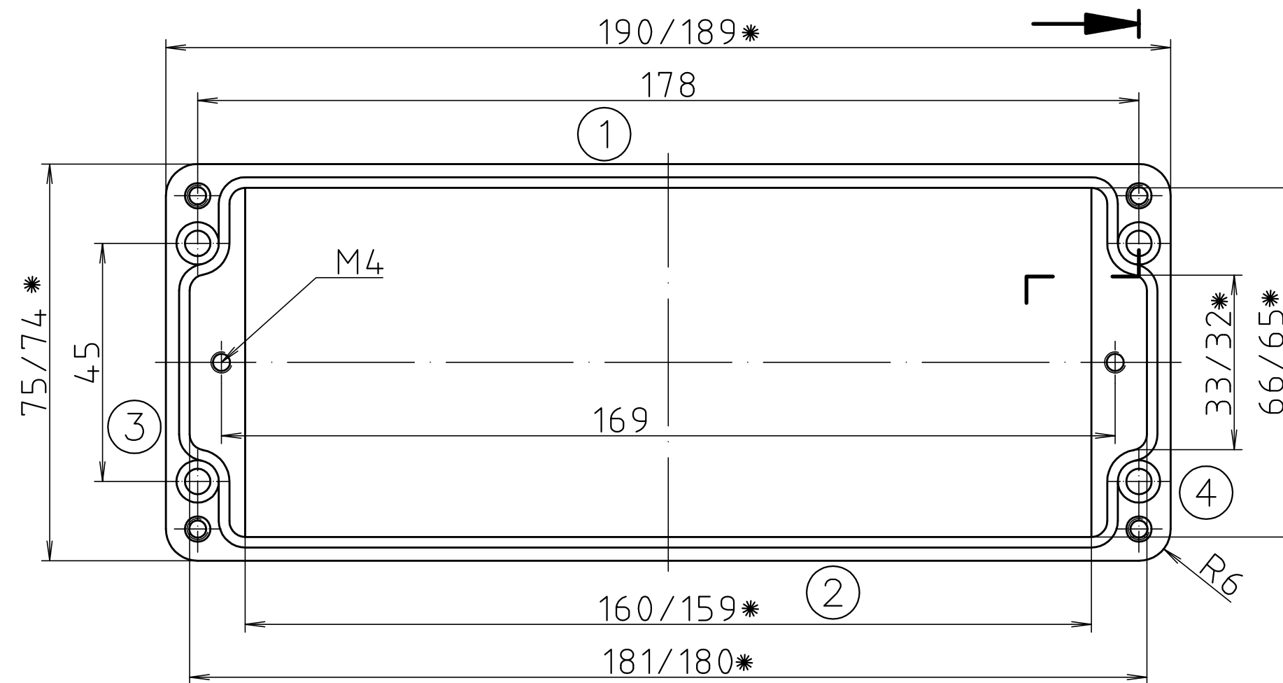
Unterteil/ base
