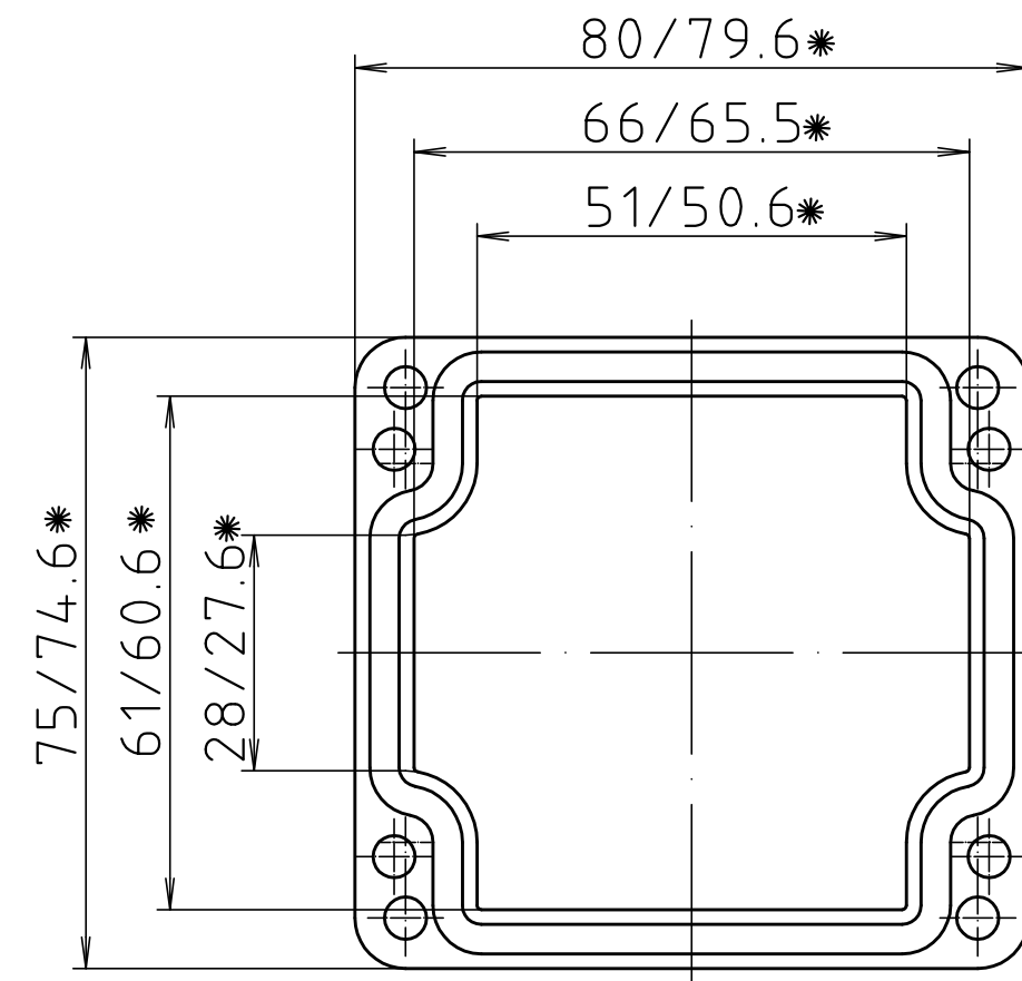
Deckel/ lid
