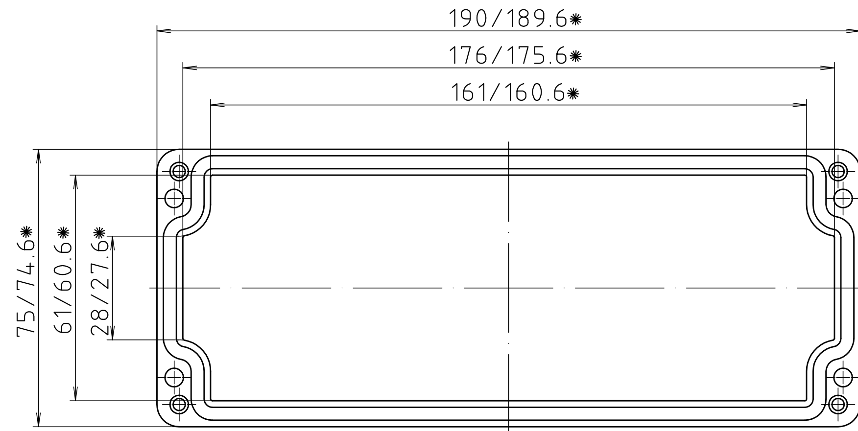
Deckel/ lid
