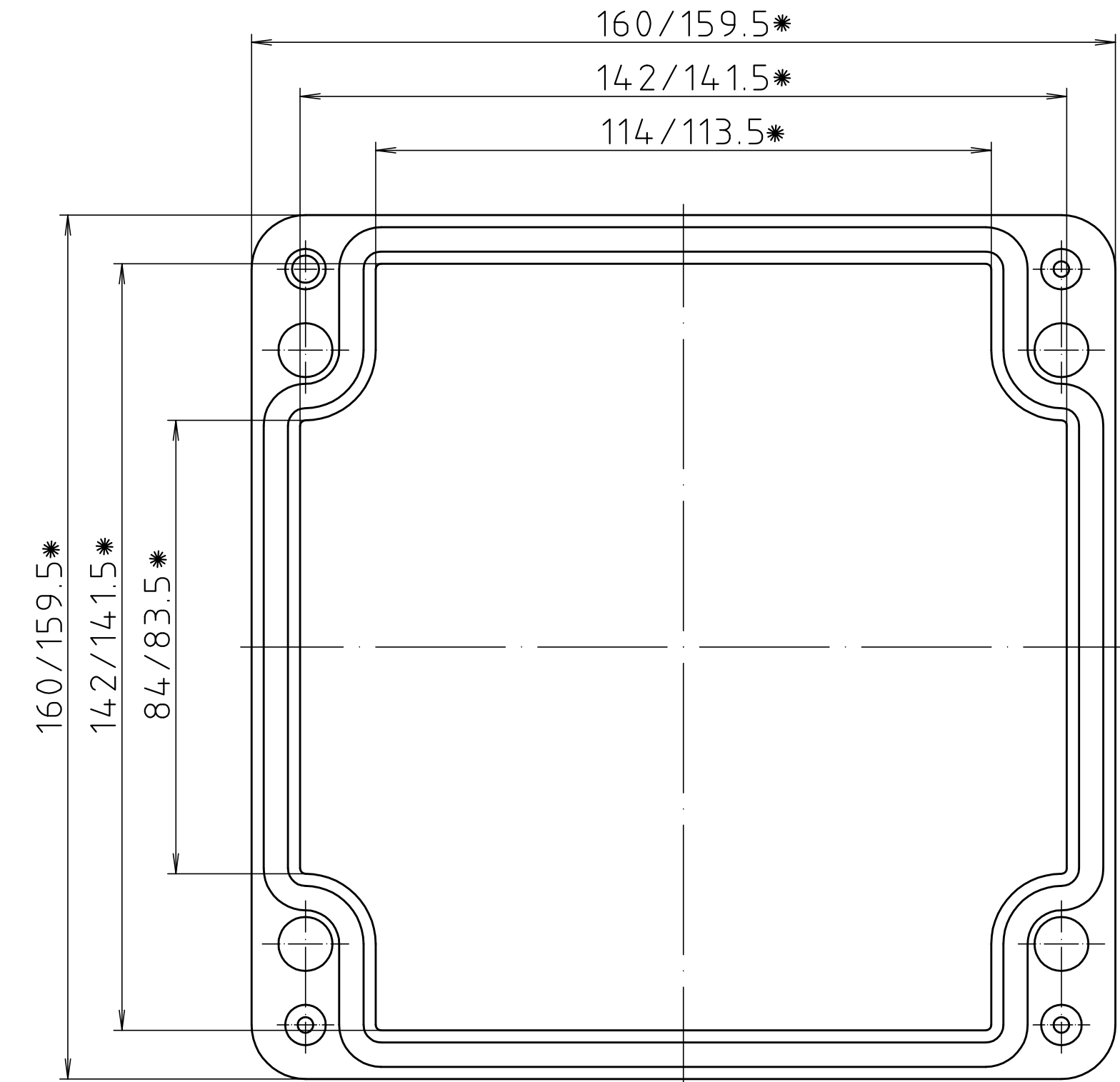
Deckel/ lid
