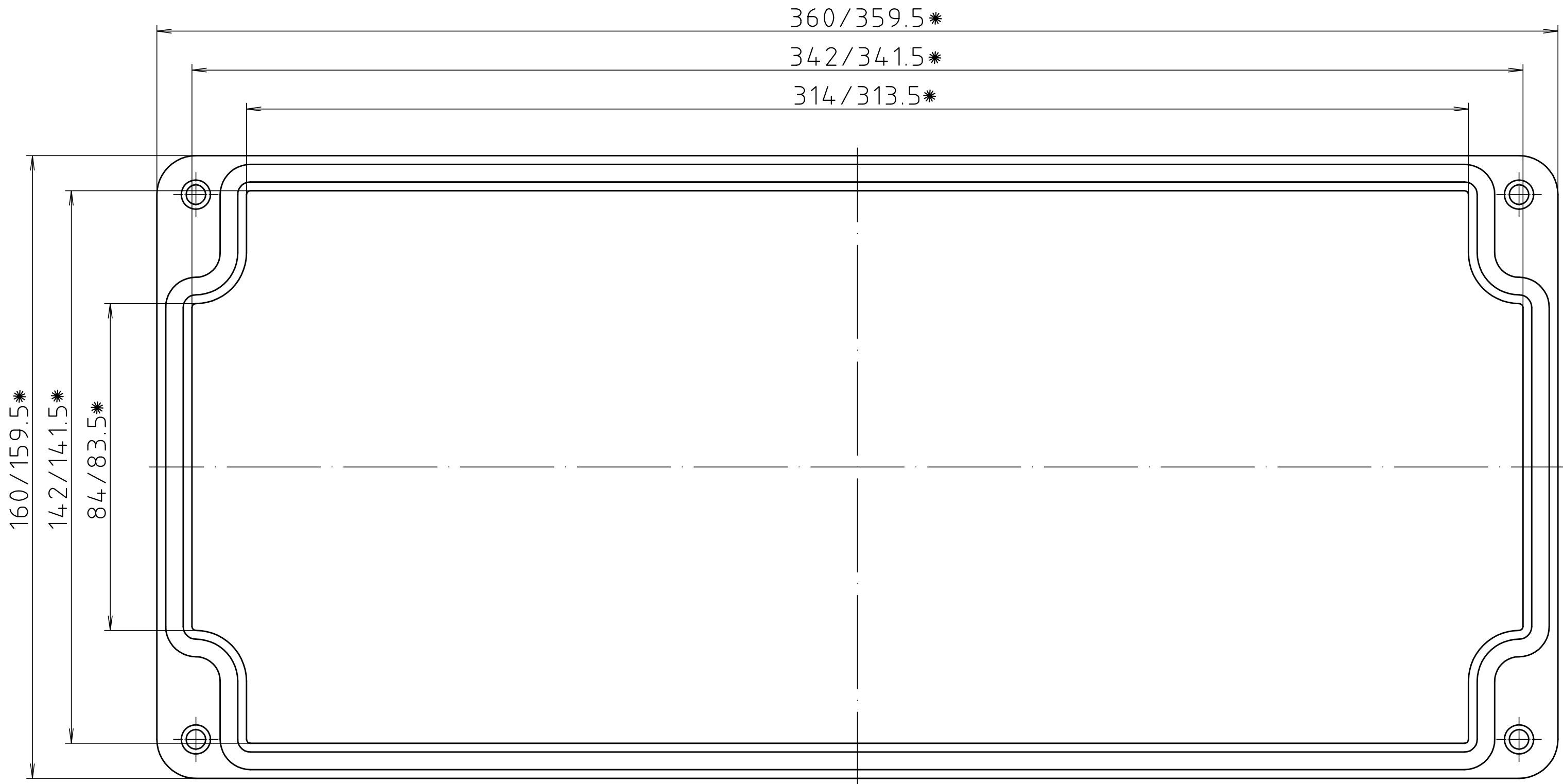
Deckel/ lid
