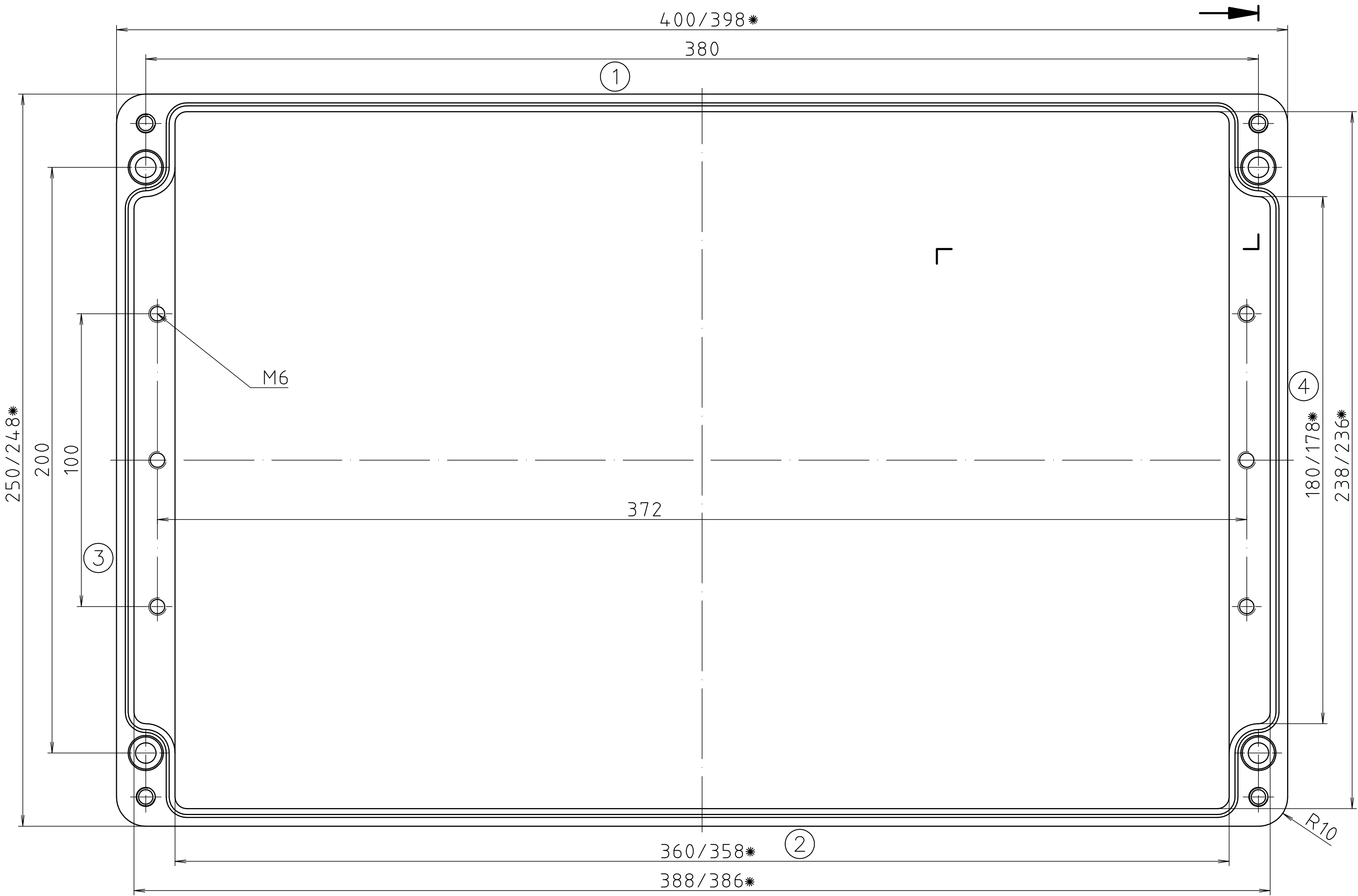
Unterteil/ base
