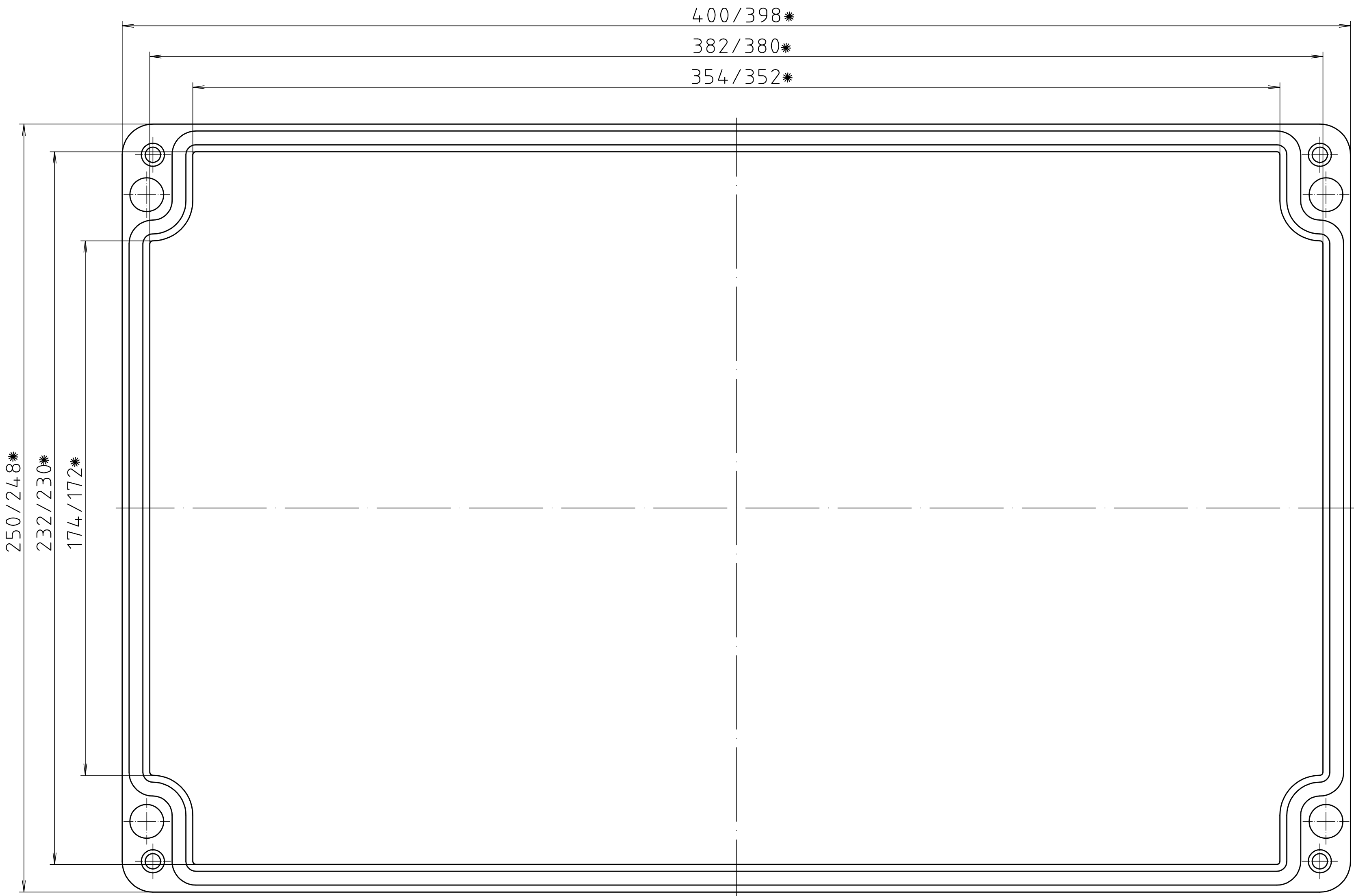
Deckel/ lid
