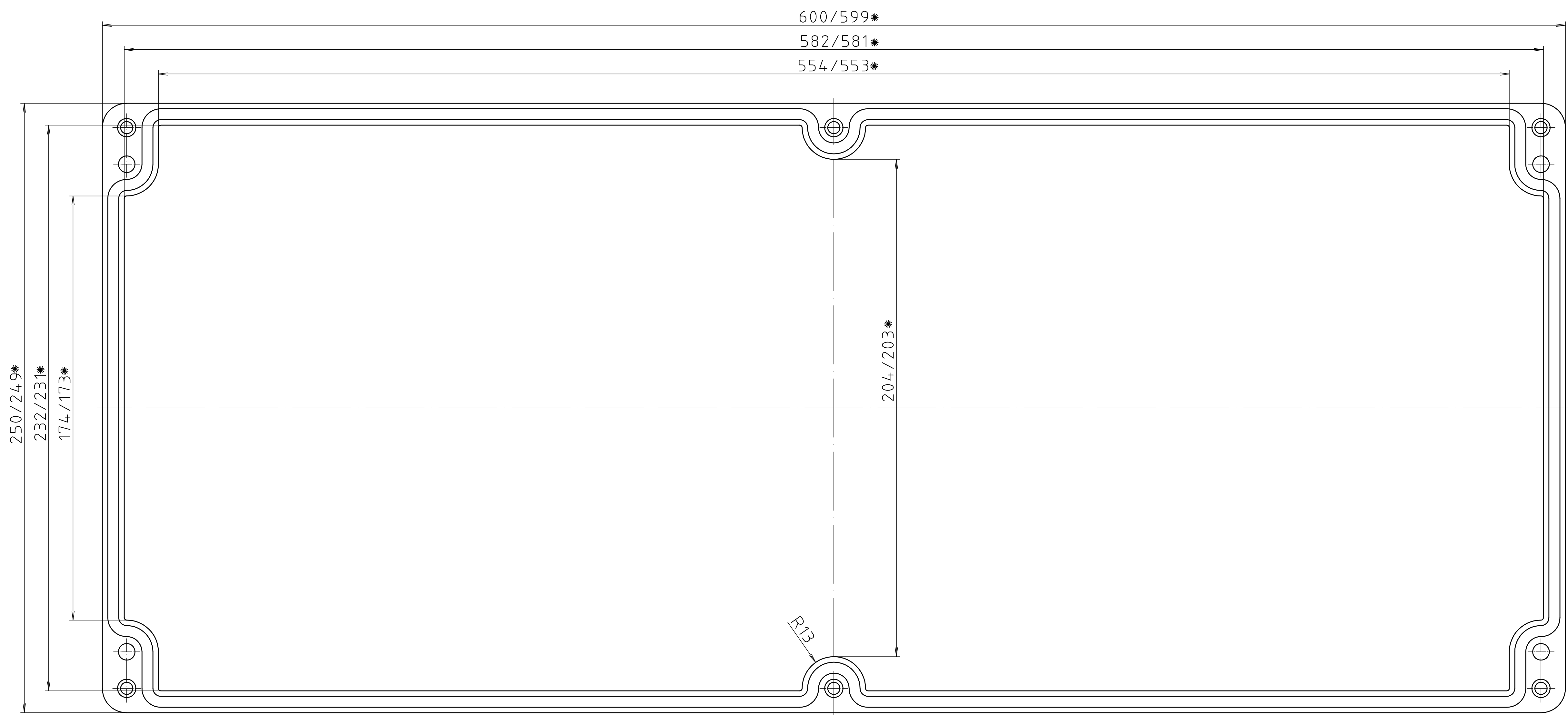
Deckel/ lid
