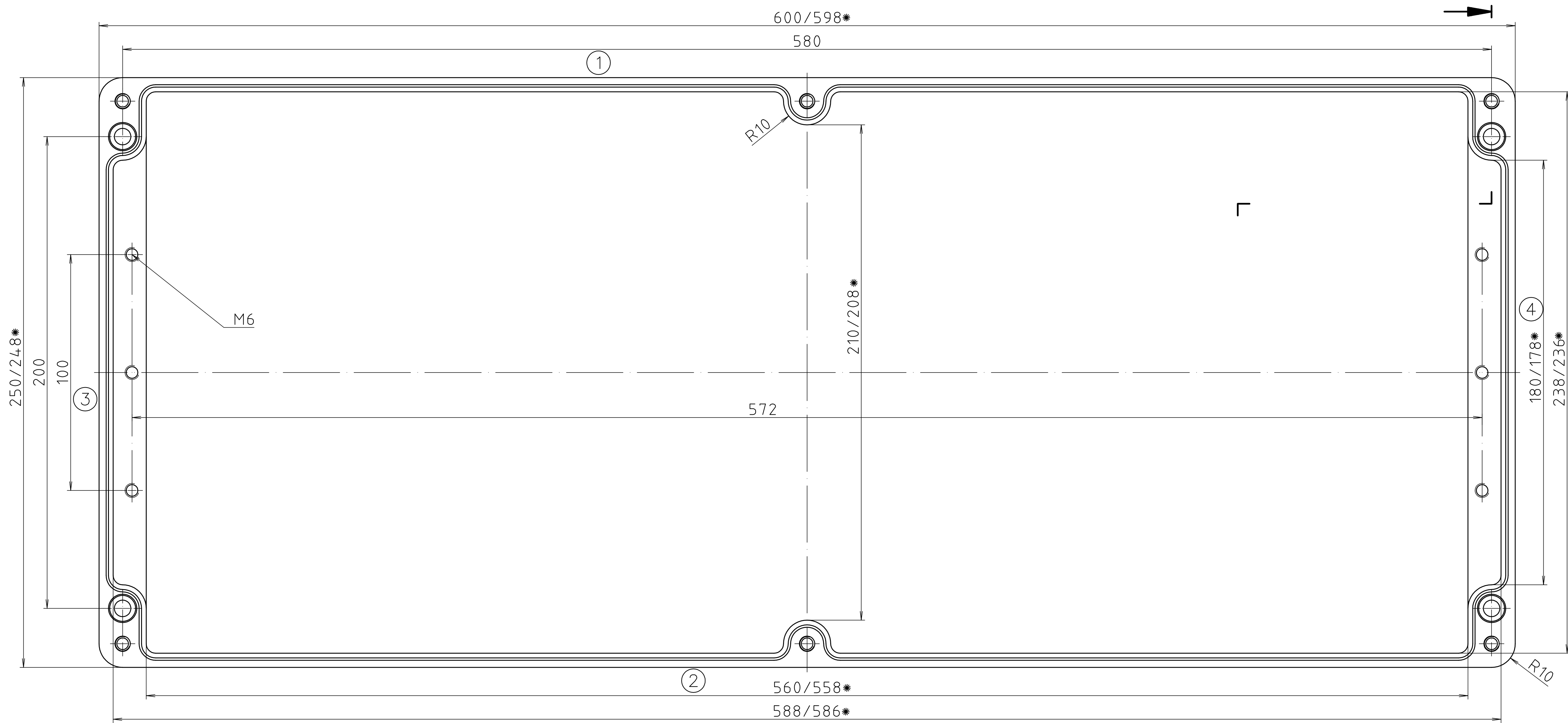
Unterteil/ base
