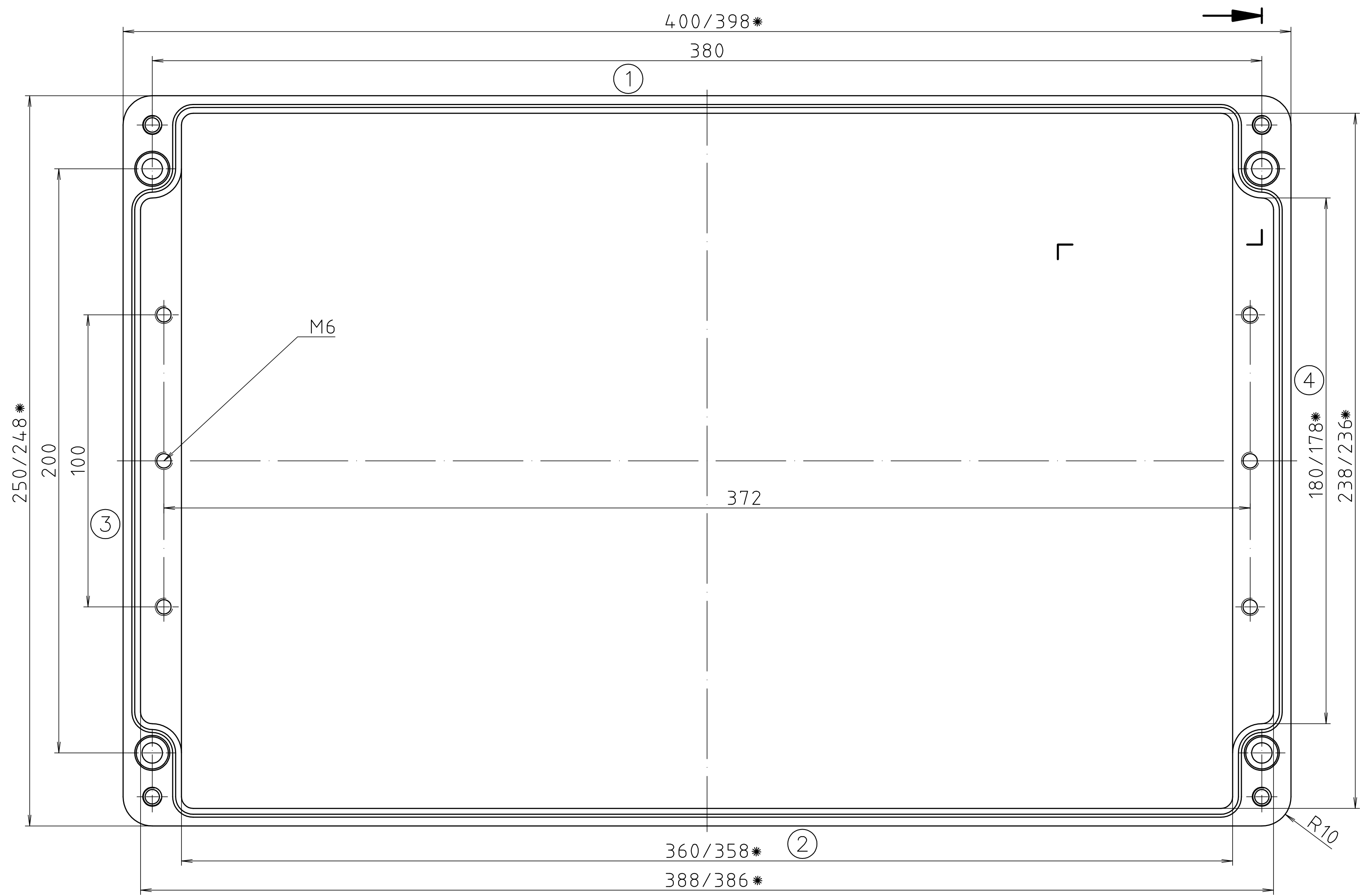
Unterteil/ base
