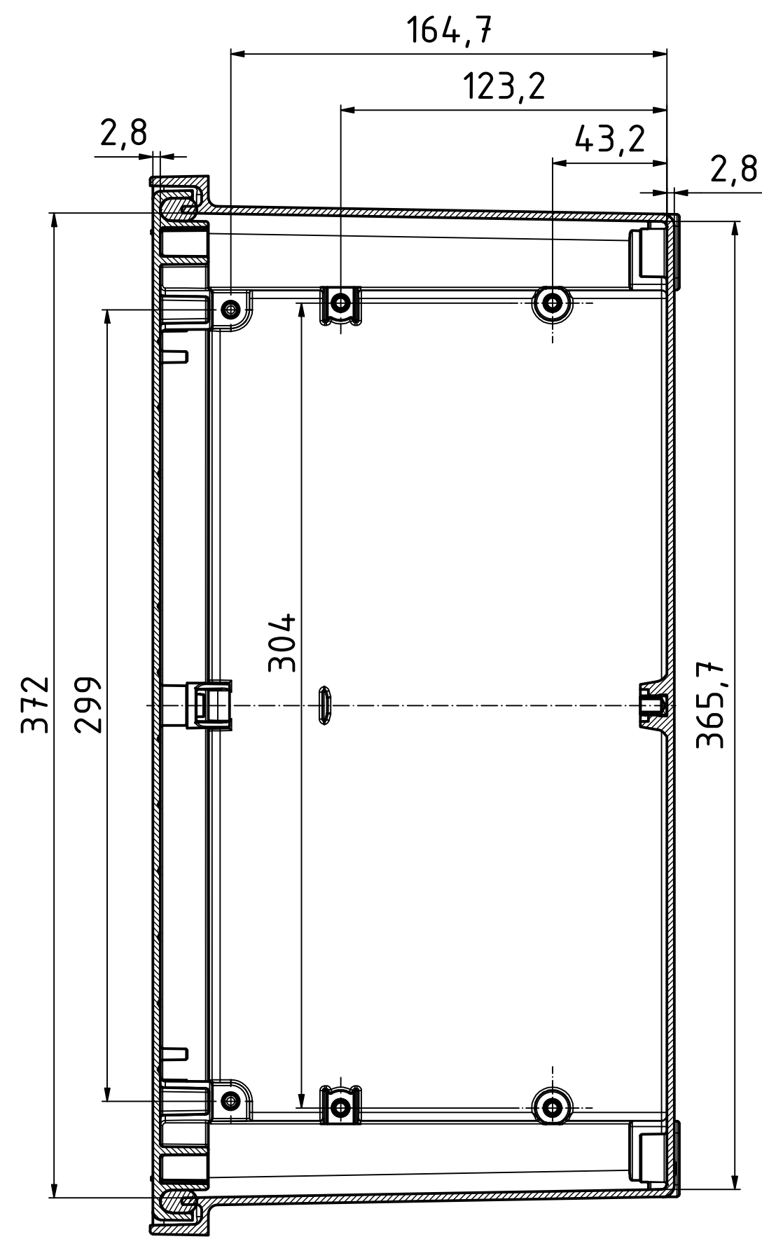
B-B ( 1 : 2 )
