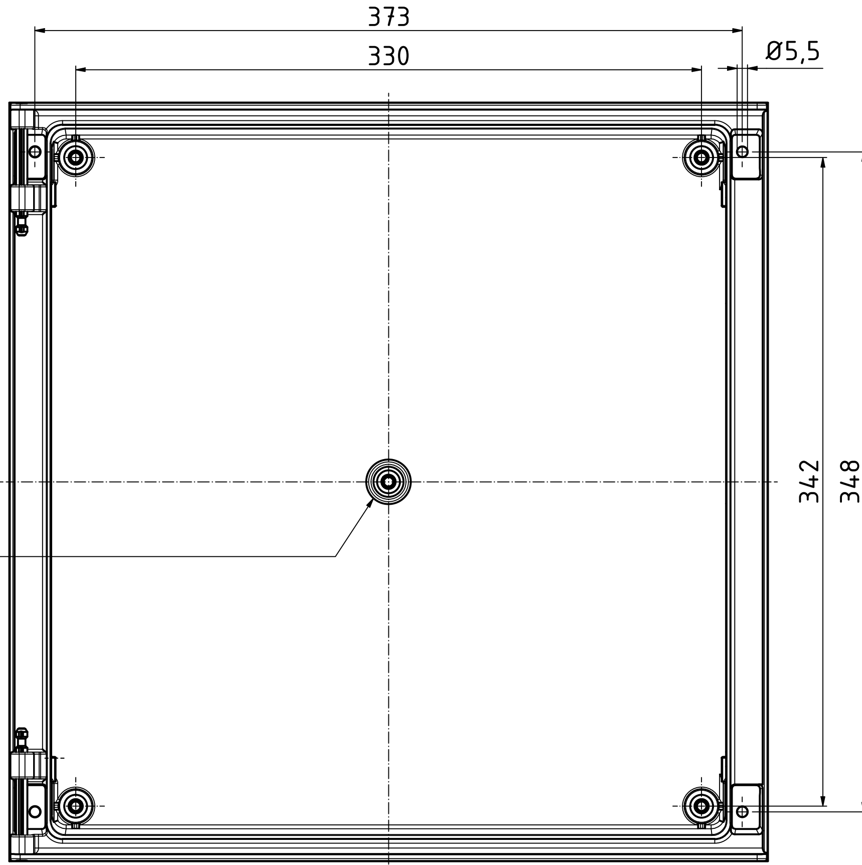
Unterteil/base ( 1 : 2 )
