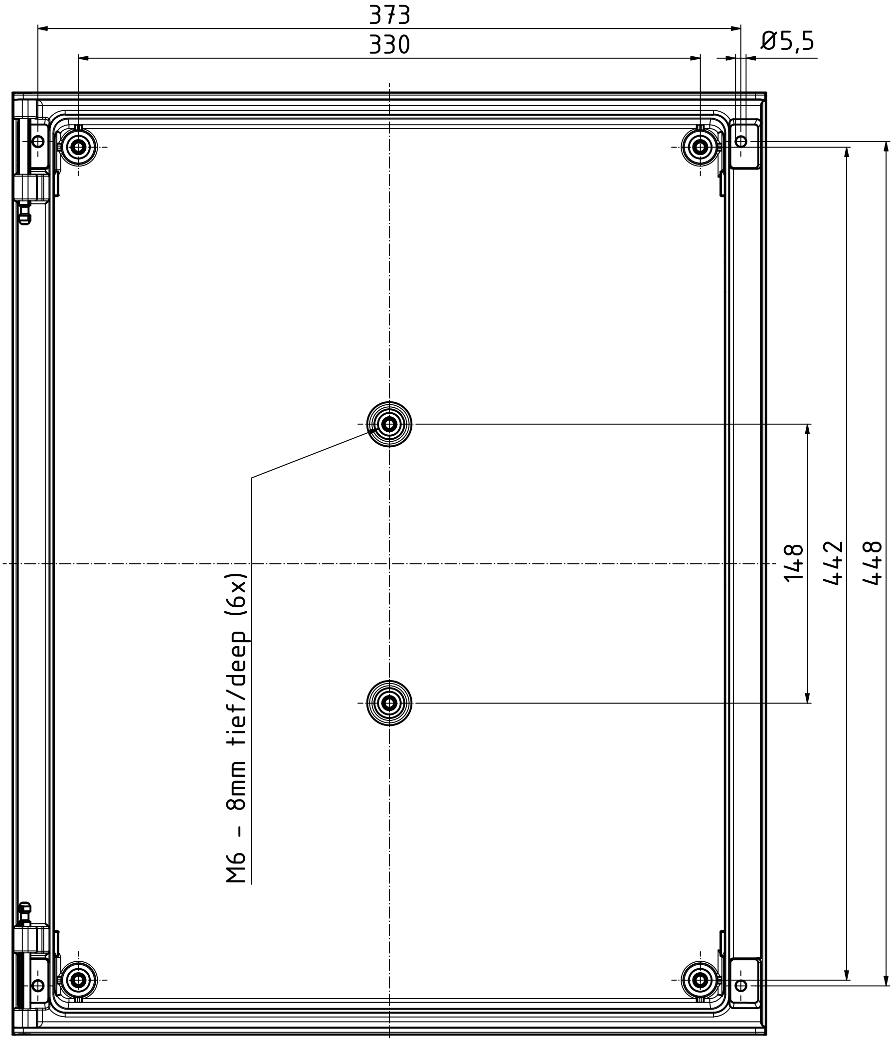
Unterteil ( 1 : 2 ) Base
